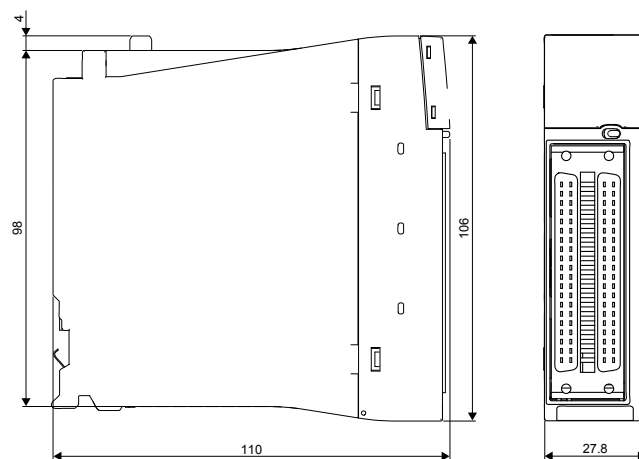
40-контактный разъем, 64-точечный модуль
