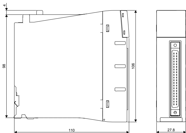
40-контактный разъем, 32-точечный модуль
