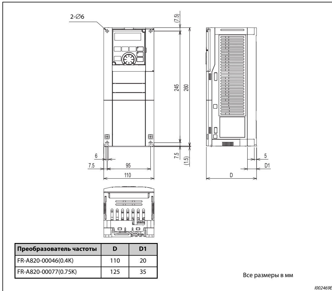
Рис. 8-1: Габаритно-присоединительные размеры преобразователей частоты FR-A820-00046(0.4K) и FR-A820-00077(0.75K)
