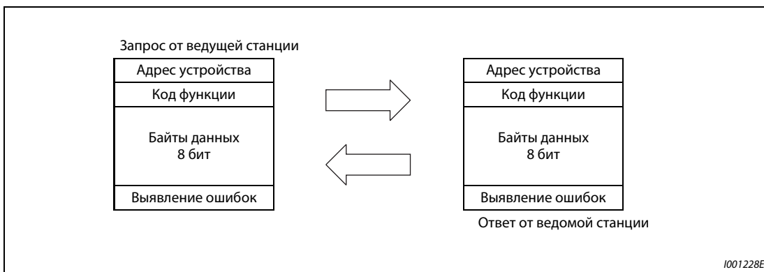
Рис. 5-305: Обмен данными
