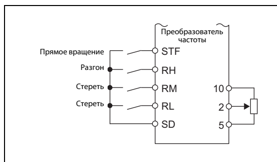
Рис. 5-93: Пример схемы для использования цифрового потенциометра
