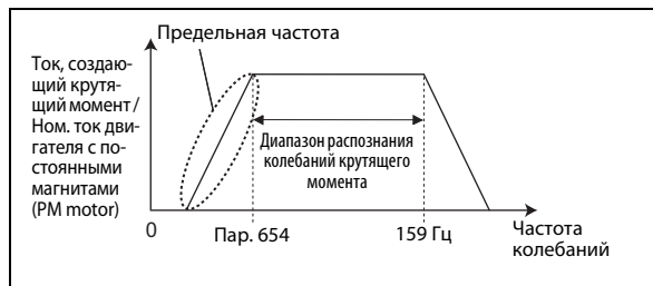
Рис. 5-338: Настройка
