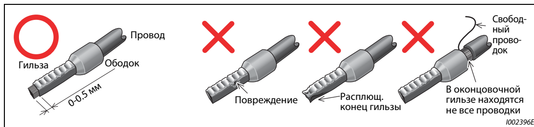
Рис. 2-28: Опрессовка оконцевочной гильзы
