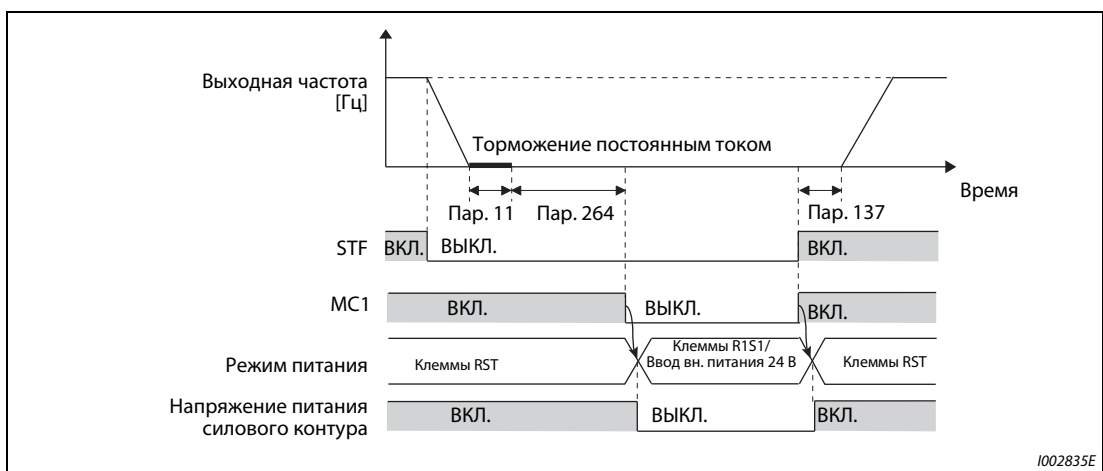
Рис. 5-219: Временная диаграмма функции автоматического уменьшения потребляемой мощности
