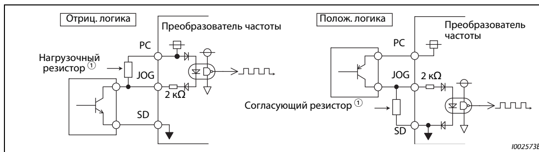
Рис. 5-107: Импульсный вход
