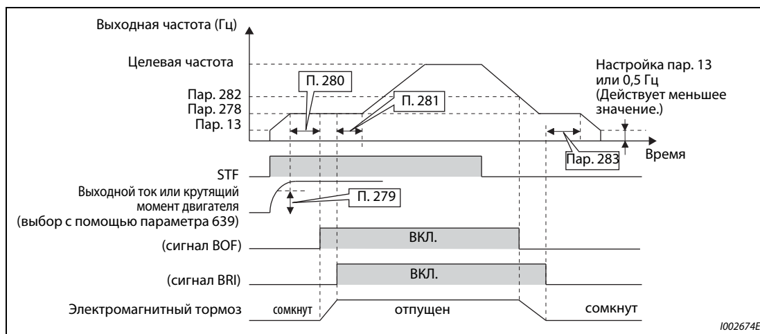
Рис. 5-221: Работа с помощью параметра 292 = 7
