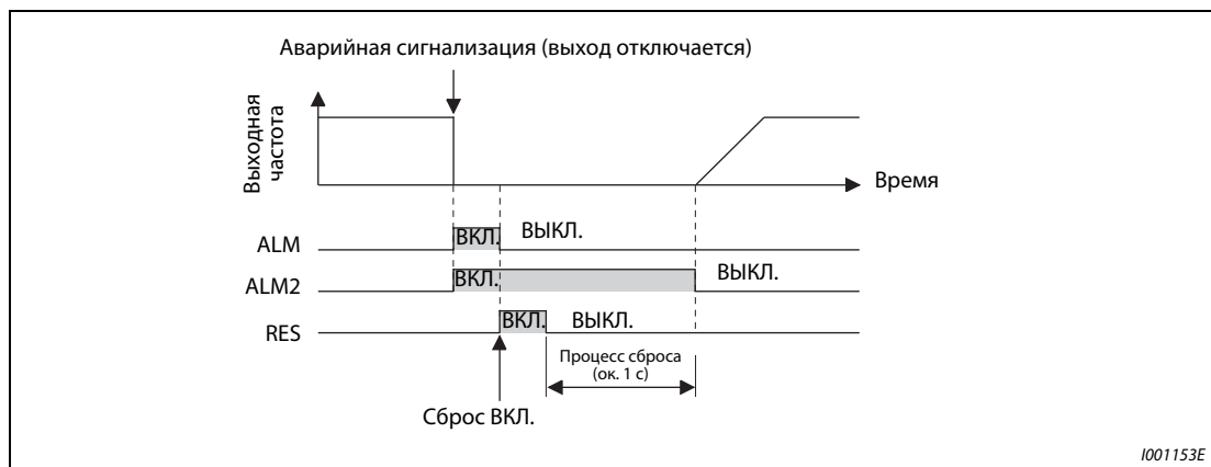
Рис. 5-162: Аварийный сигнал
