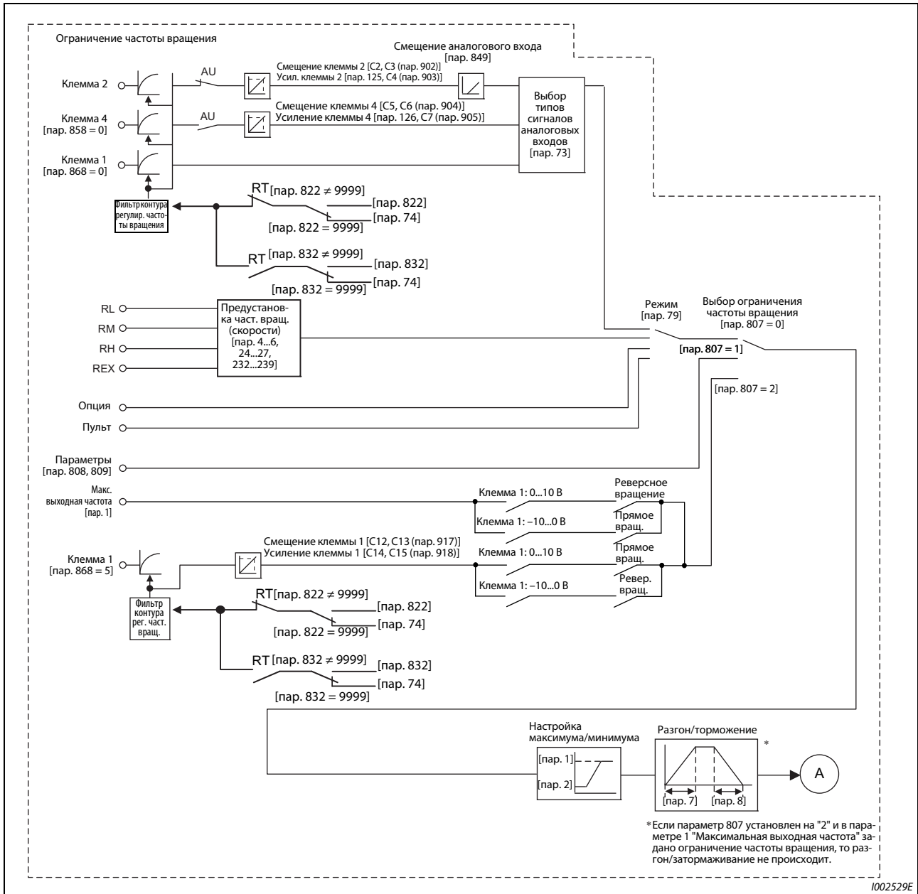
Рис. 5-36: Блок-схема
