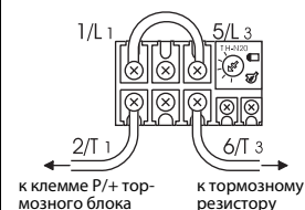
Таб. 2-44: Сочетание тормозного резистора G(R)ZG и термовыключателя
