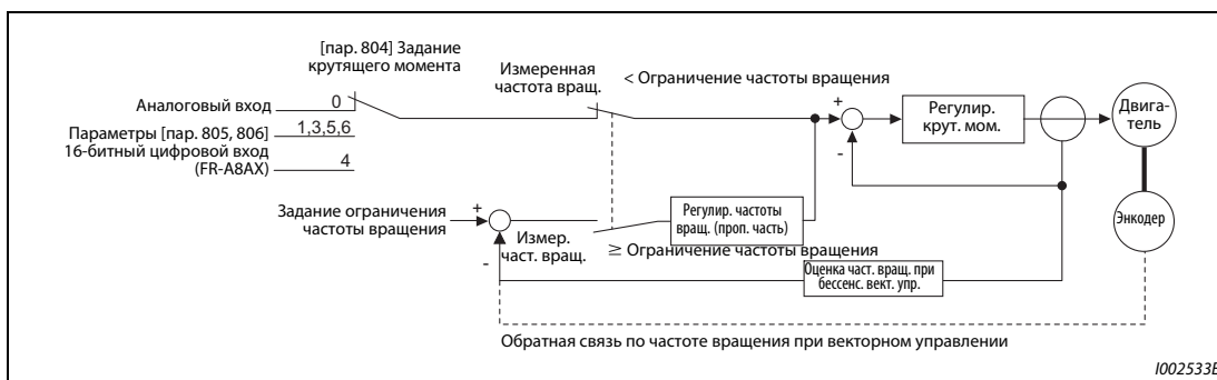
Рис. 5-40: Блок-схема
