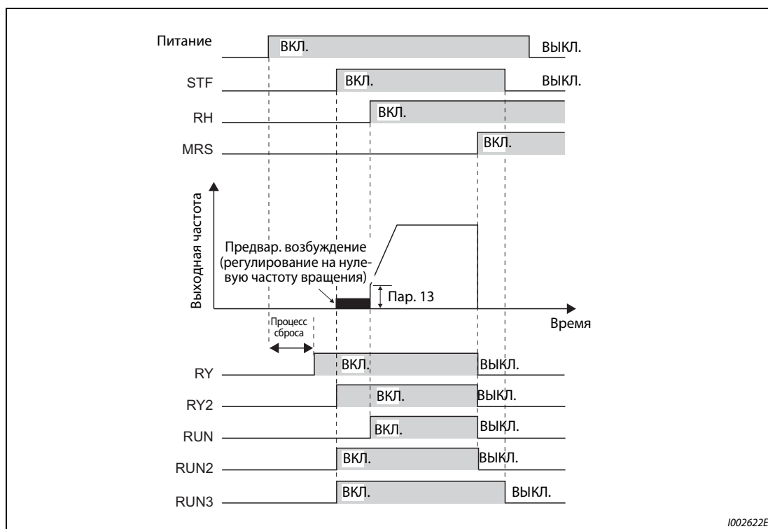
Рис. 5-159: Готовность к работе и вращение двигателя
