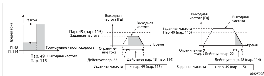
Рис. 5-136: Примеры настройки предельного тока
