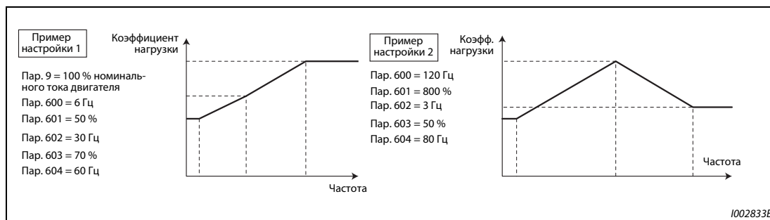
Fig. 5-124: Примеры настройки
