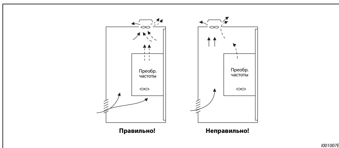
Рис. 2-14: Расположение преобразователя в шкафу с направленным движением воздуха
