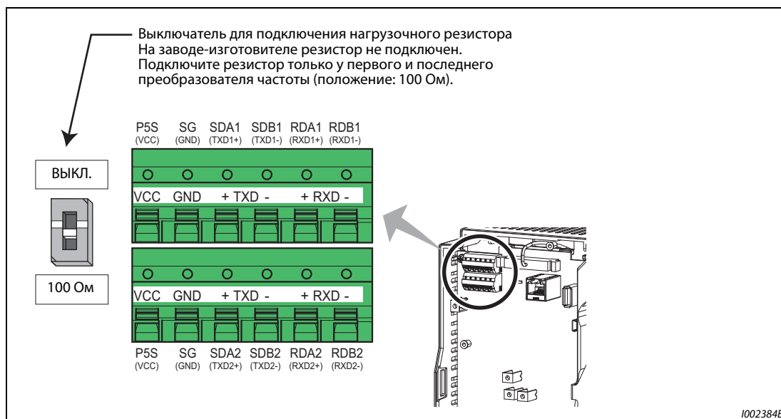
Рис. 2-43: 2-й последовательный интерфейс преобразователя частоты
