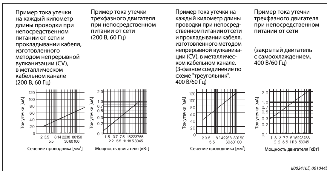
Рис. 3-2: Токи утечки
