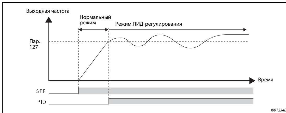
Рис. 5-252: Автоматическое переключение в режим ПИД-регулирования
