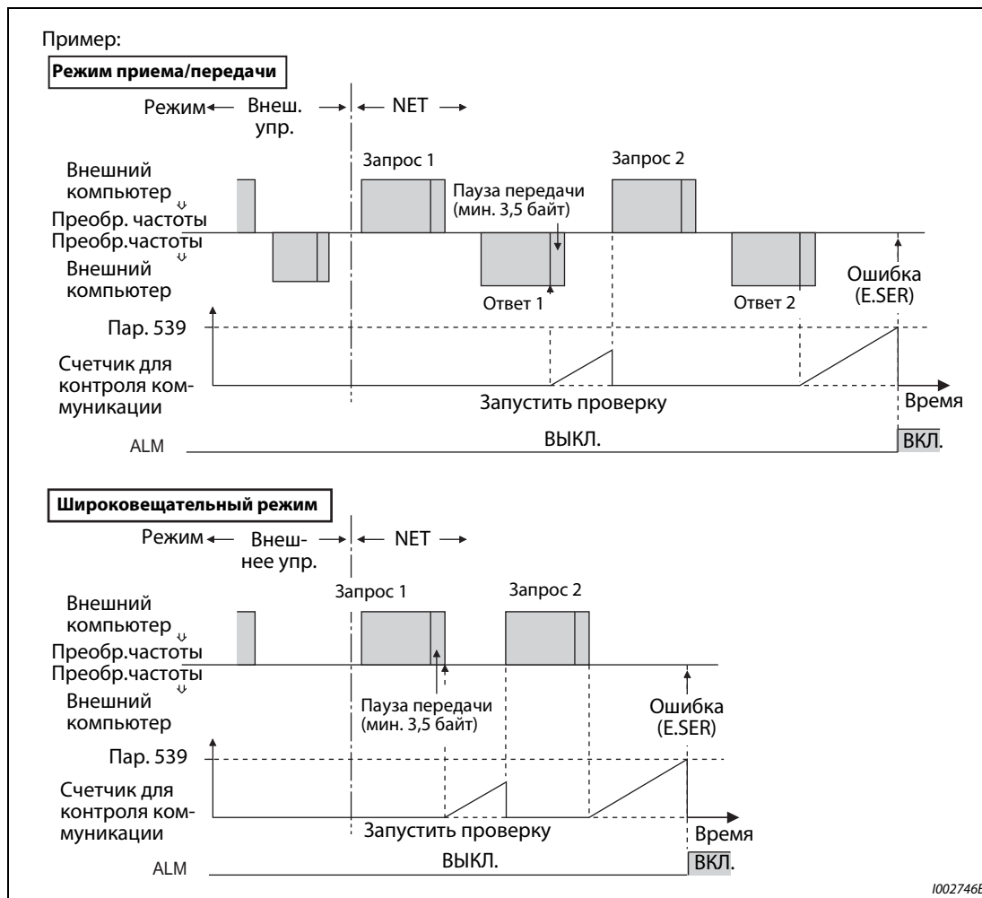
Рис. 5-307: Контроль на обрыв кабеля
