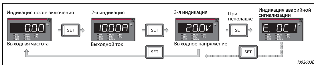
Рис. 5-139: Индикация различных рабочих величин
