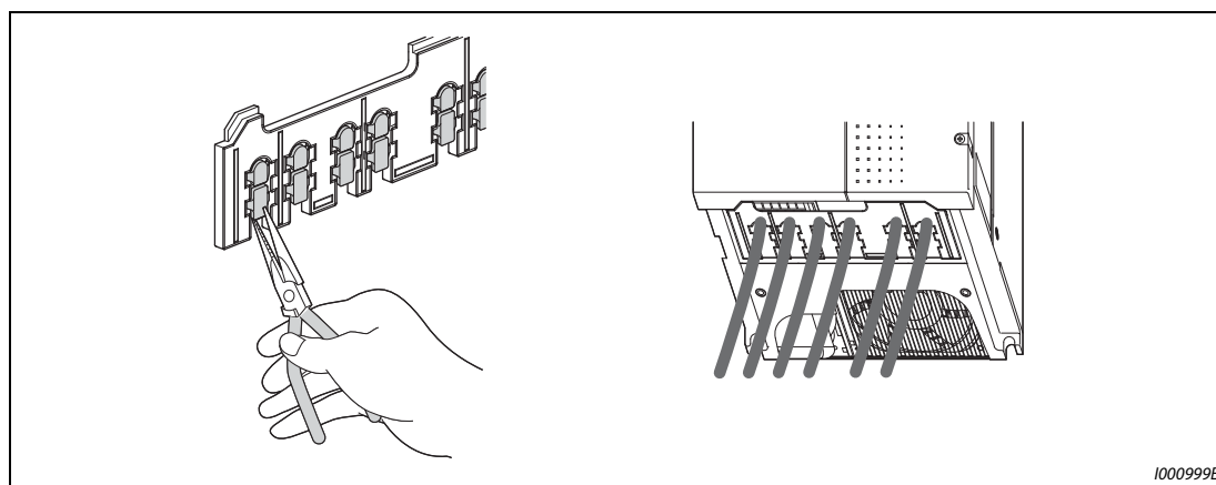
Рис. 2-19: Гребенка для ввода кабелей
