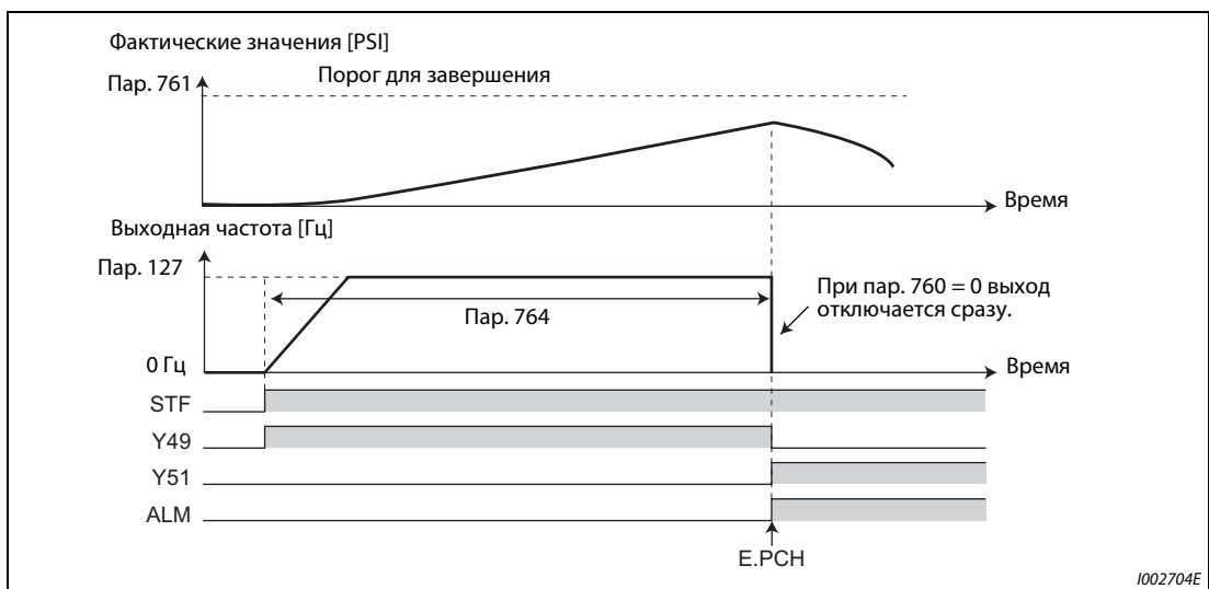
Рис. 5-261: Достижение предела времени при режиме предварительного заполнения
