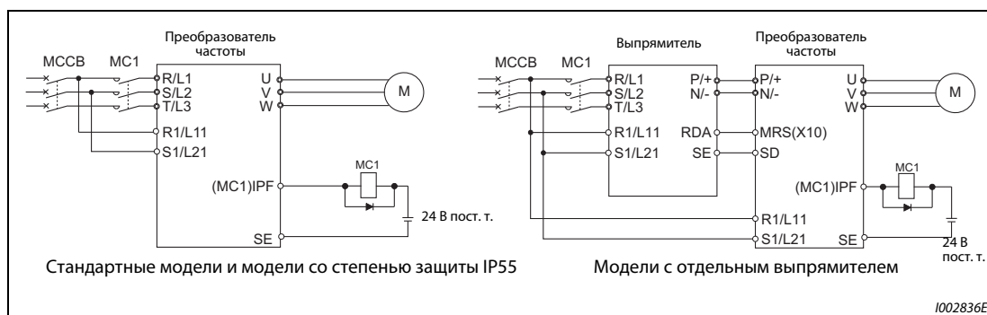
Рис. 5-217: Электропитание через клеммы R1 и S1
