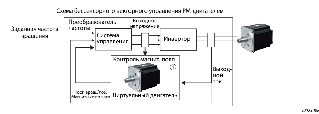
Рис. 5-1: Схема бессенсорного векторного управления PM-двигателем
