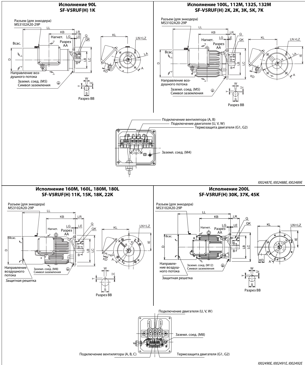
Рис. 8-12: Габаритно-присоединительные размеры двигателей SF-V5RUF(H) (с крепежным фланцем)
