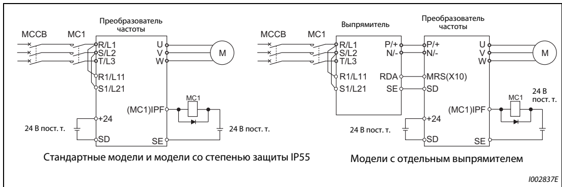
Рис. 5-218: Питание от внешнего источника 24 В
