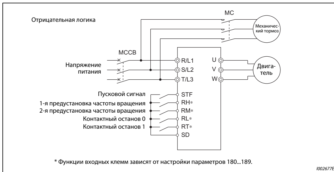
Рис. 5-224: Пример подключения
