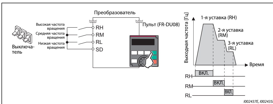
Рис. 4-5: Вызов установки частоты вращения (скорости) с помощью выключателя
