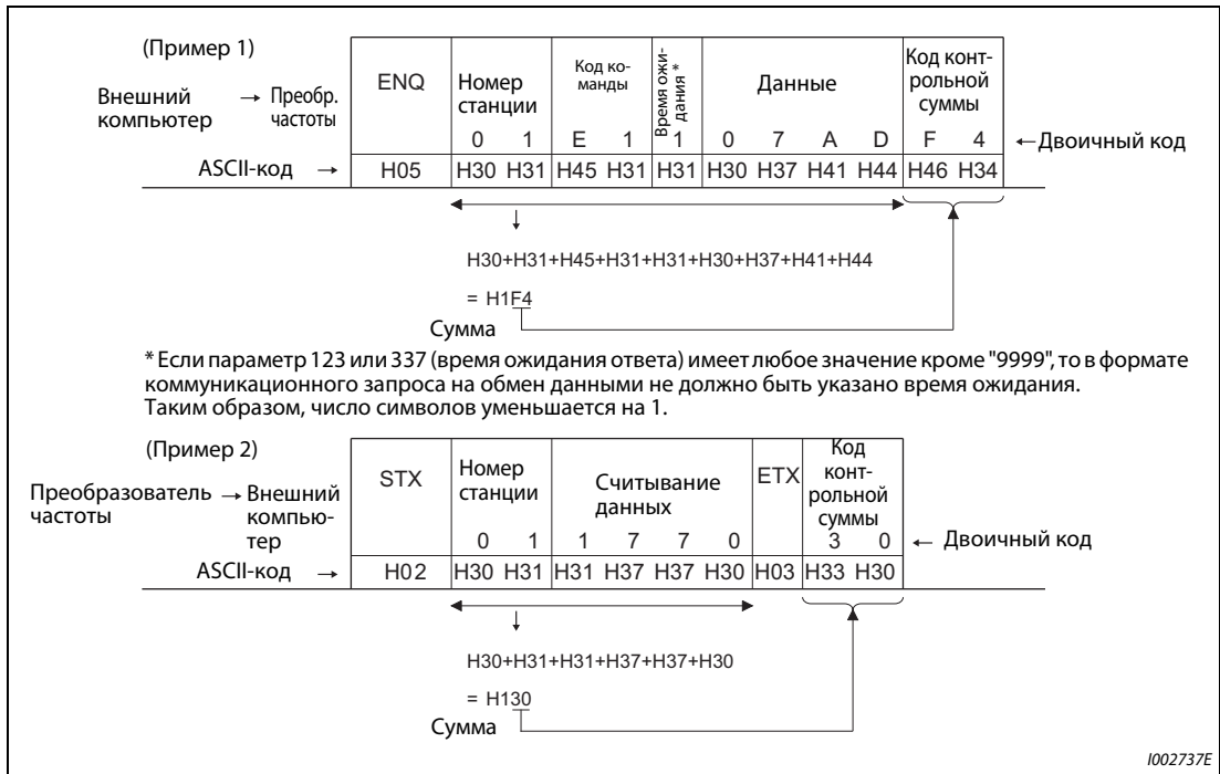
Рис. 5-299: Код контрольной суммы (примеры)
