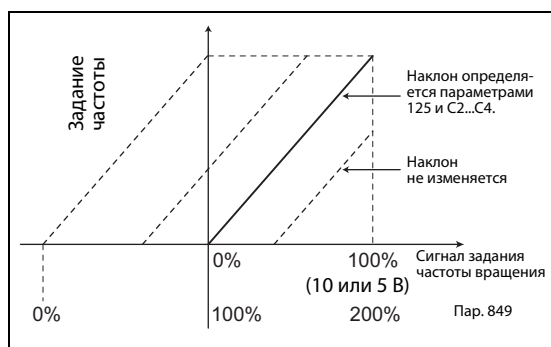
Рис. 5-189: Настройка смещения
