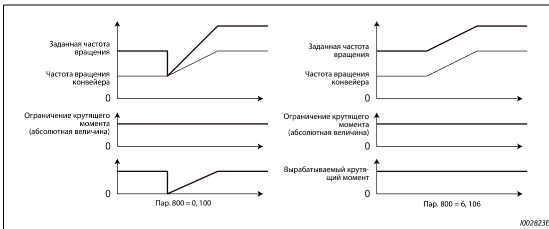
Рис. 5-52: Выбатываемый крутящий момент в зависимости от параметра 800
