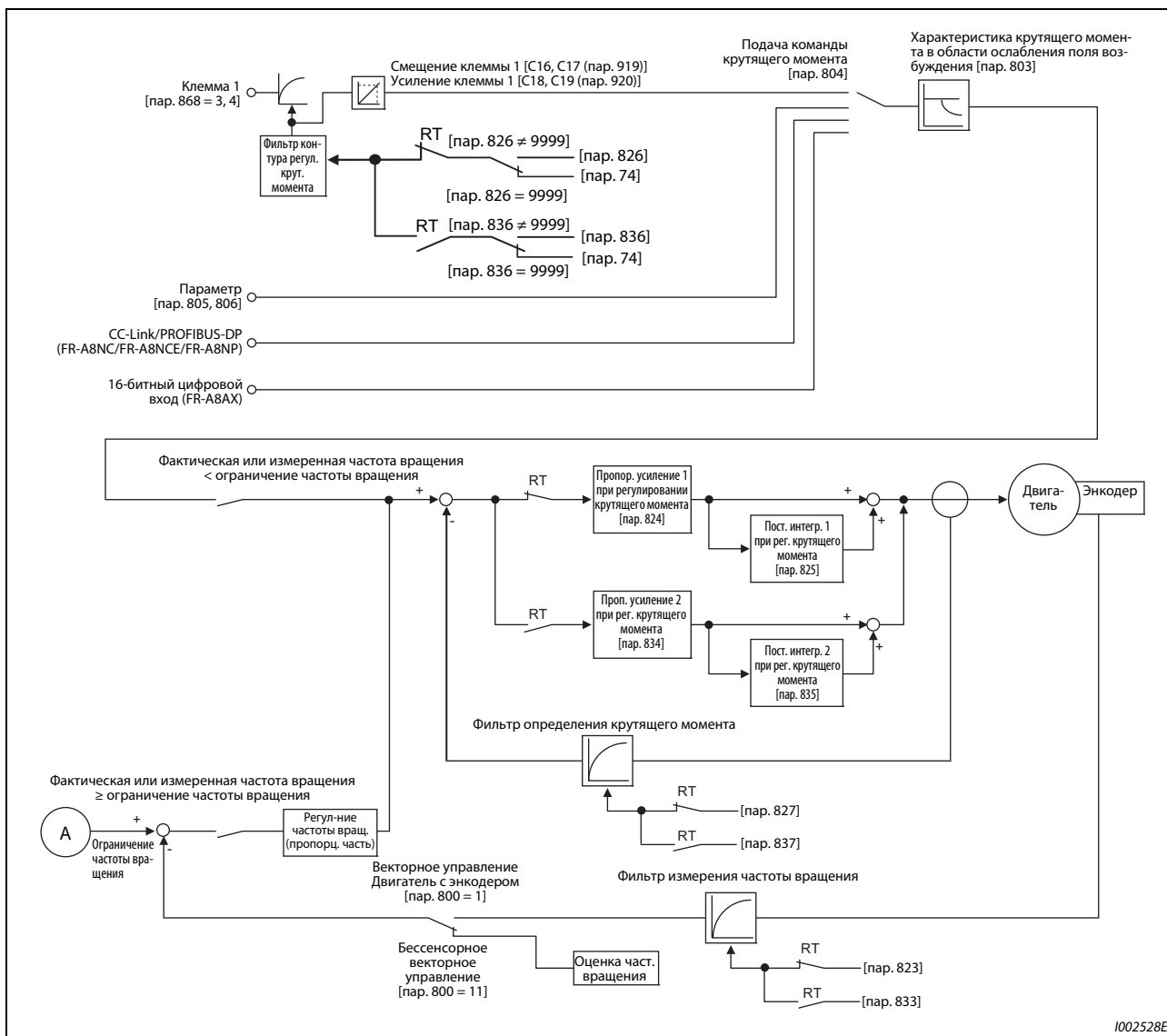
Рис. 5-35: Блок-схема
