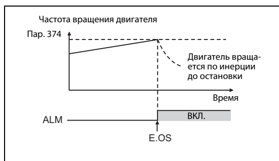
Рис. 5-138: Предел частоты вращения и вывод аварийной сигнализации
