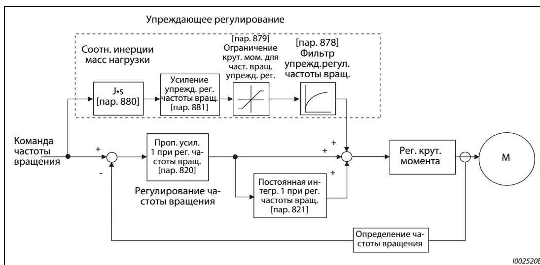
Рис. 5-27: Блок-схема упреждающего регулирования
