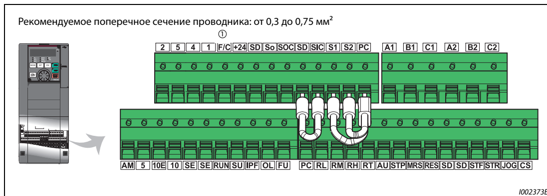
Рис. 2-30: Клеммы управляющего контура
