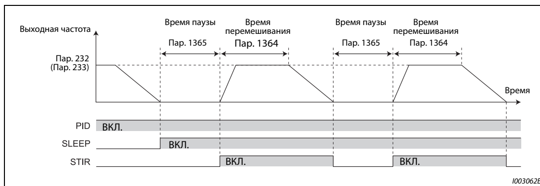
Рис. 5-196: Режим перемешивания в ПИД-состоянии SLEEP
