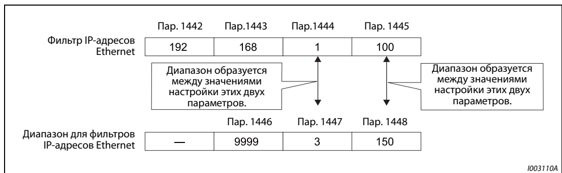
Рис. 5-251: Пример 1 настройки для фильтрации IP-адресов Ethernet
