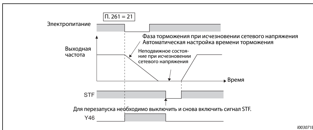
Рис. 5-217: Автоматическая настройка времени торможения
