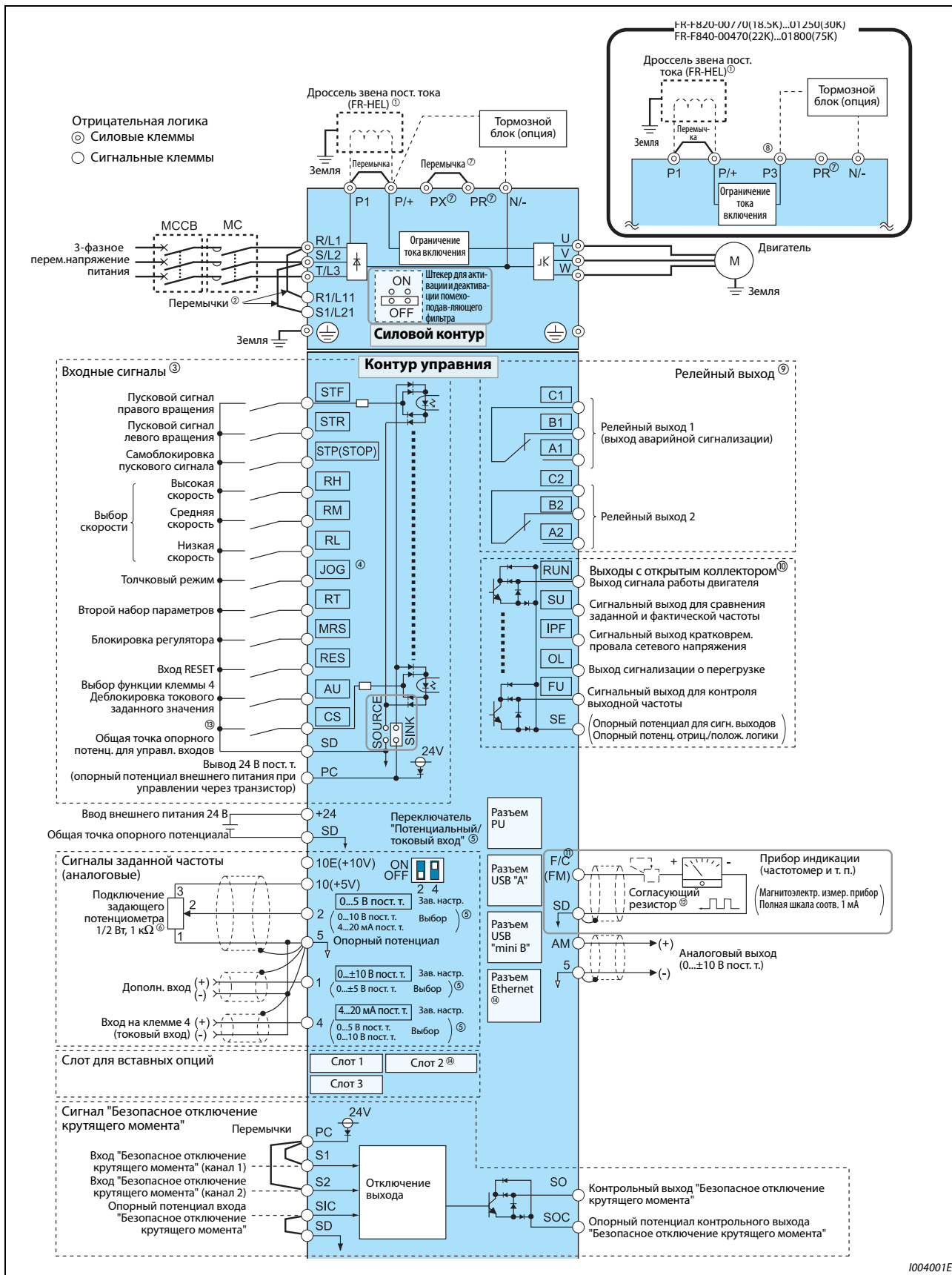
Рис. 2-22: Схема подключения преобразователя частоты (тип FM) (FR-F800-E)
