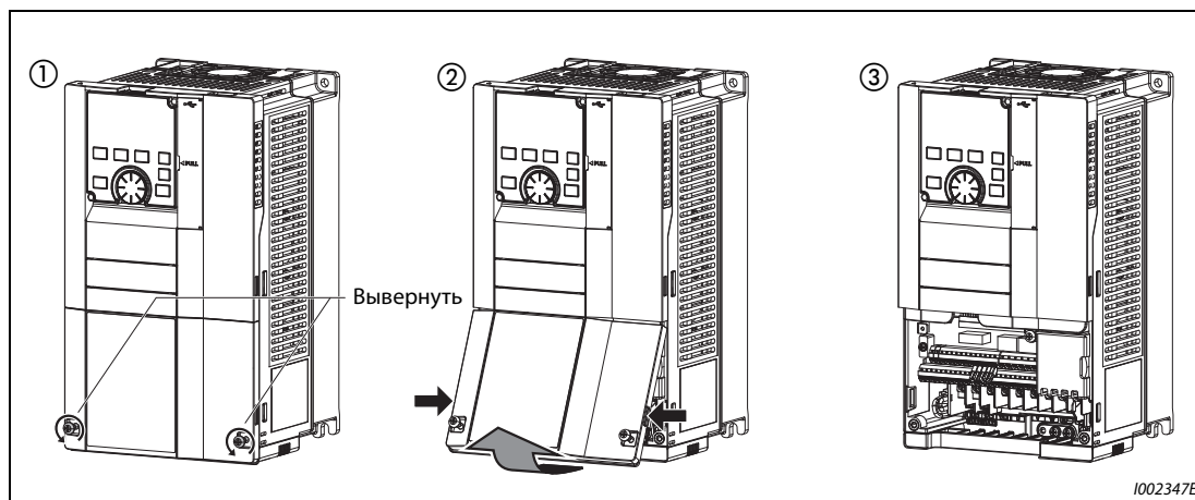
Рис. 2-7: Снятие нижней передней панели
