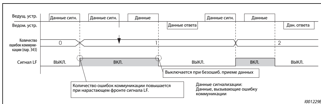
Рис. 5-244: Вывод сигнала LF
