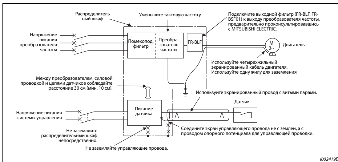
Рис. 3-6: Примеры подавления помех
