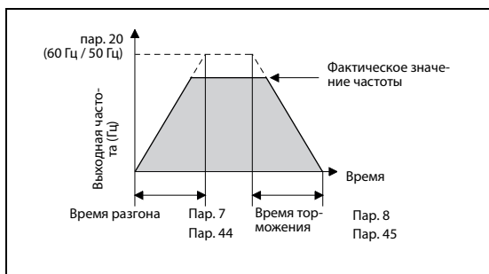
Рис. 5-17: Время разгона/торможения
