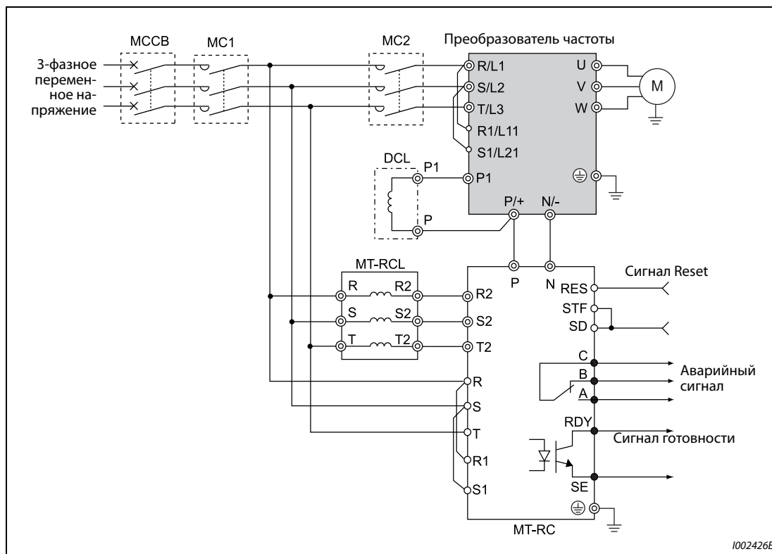
Рис. 2-55: Подключение блока рекуперации (MT-RC)
