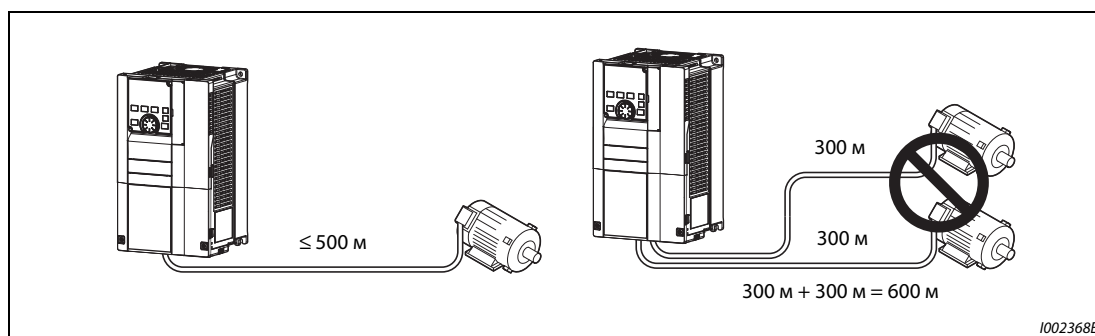
Рис. 2-24: Общая длина проводки (FR-F820-00105(2.2K) и выше, FR-F840-00052(2.2K) и выше)
