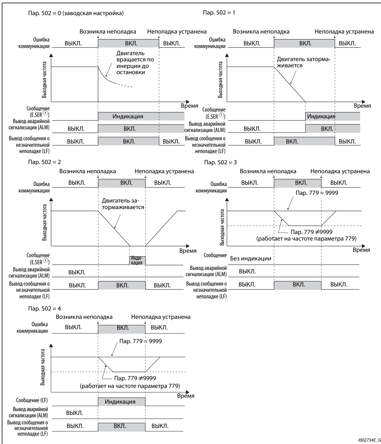
Рис. 5-231: Характер работы при ошибке коммуникации
