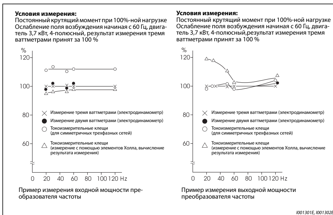
Рис. 7-12: Различные методы измерения мощности дают различные результаты
