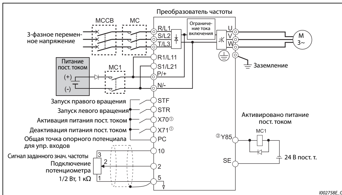
Рис. 5-272: Пример подключения для варианта 2 питания контура постоянного тока
