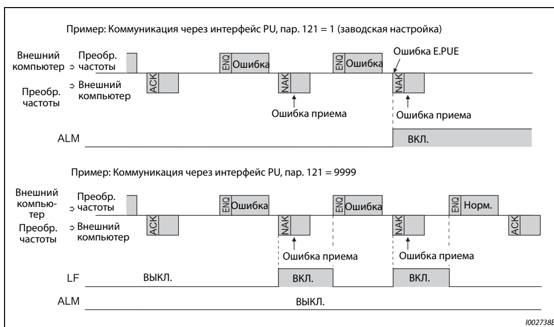
Рис. 5-239: Ошибка передачи данных
