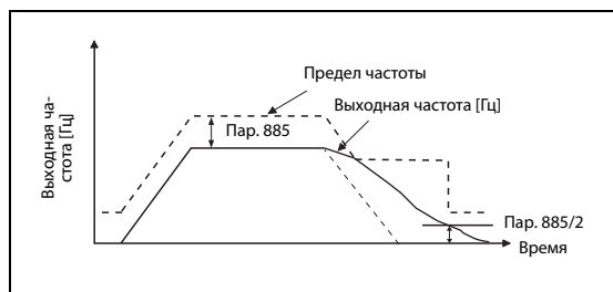
Рис. 5-277: Ограничение выходной частоты
