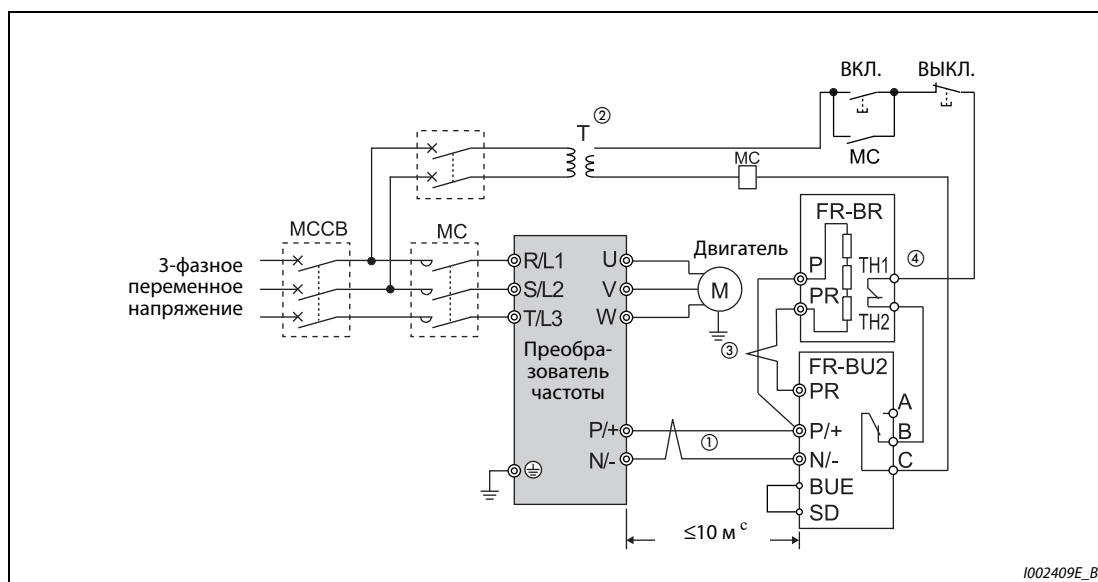
Рис. 2-49: Подключение тормозного блока с тормозным резистором FR-BR(-H)
