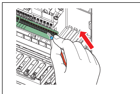
Рис. 2-33: Подсоединение провода
