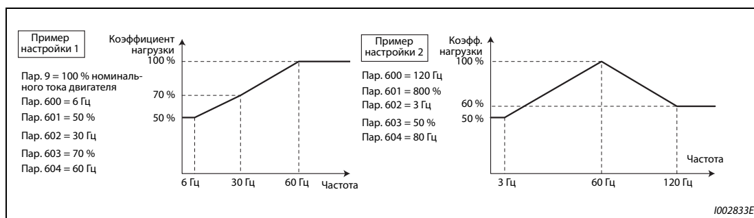
Рис. 5-55: Примеры настройки
