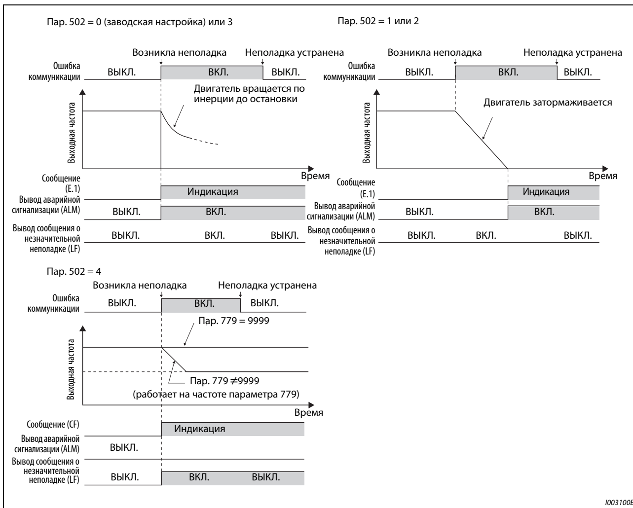
Рис. 5-232: Характер работы при ошибке коммуникационной опции
