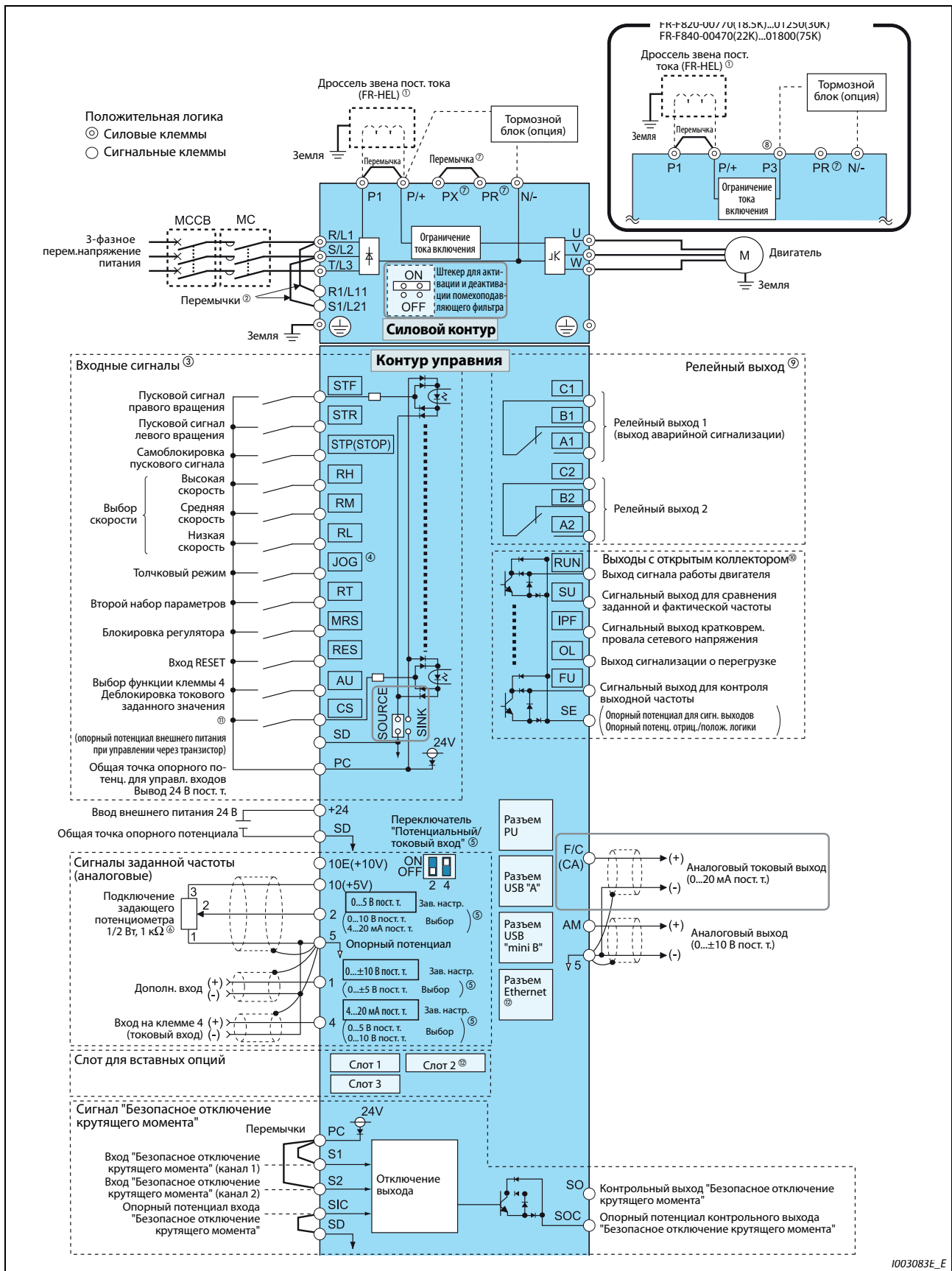
Рис. 2-21: Схема подключения преобразователя частоты (тип CA) (FR-F800-E)
