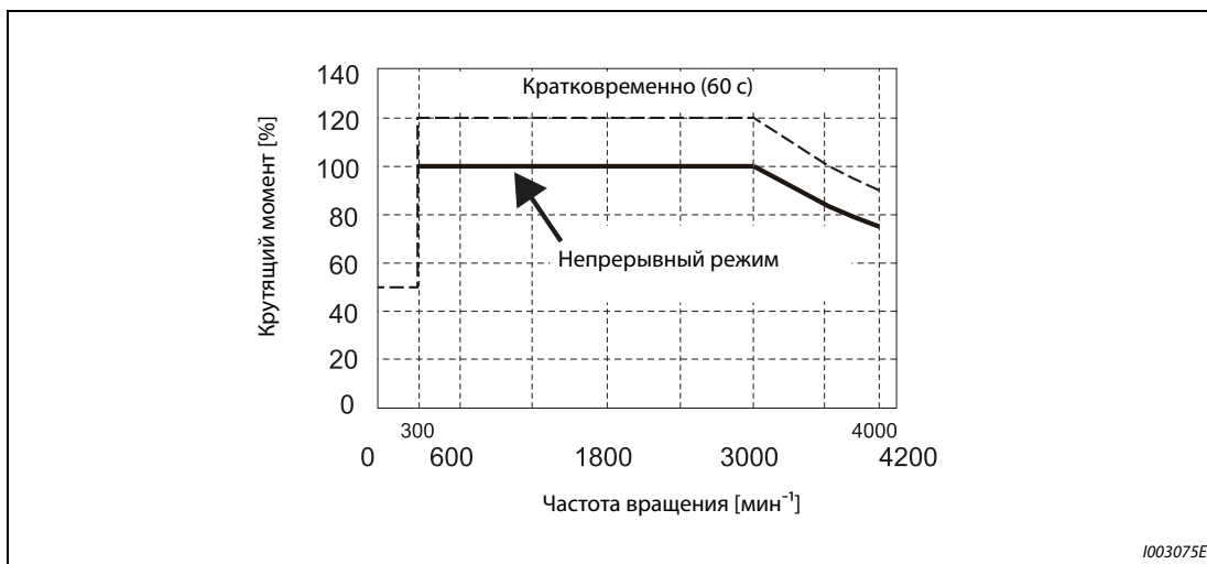
Рис. 8-2: Характеристика крутящего момента двигателей [ММ-EFS (ном. частота вращения 3000 мин -1 )]
