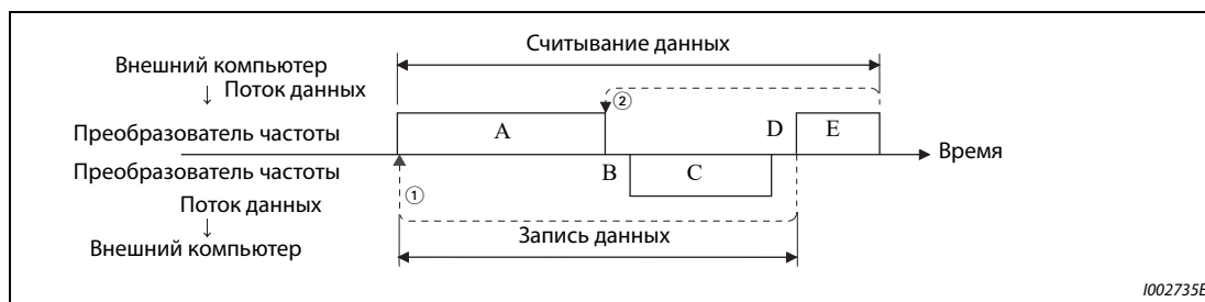
Рис. 5-235: Схематическое изображение обмена данными
