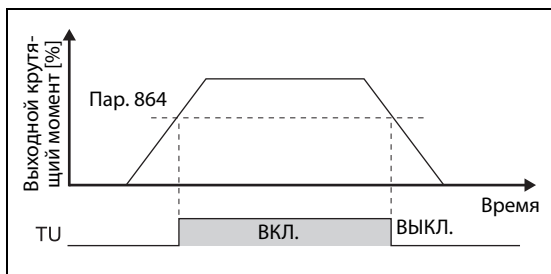
Рис. 5-103: Контроль крутящего момента
