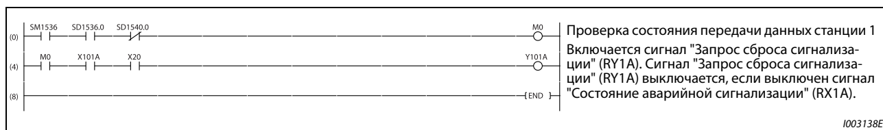
Рис. 5-298: Пример программы 9
