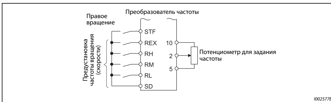
Рис. 5-43: Пример подключения
