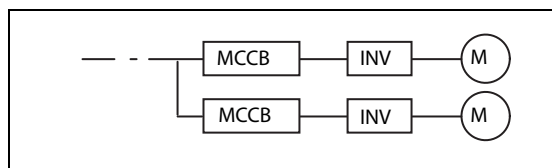
Рис. 2-4: Компоновка силовых выключателей
