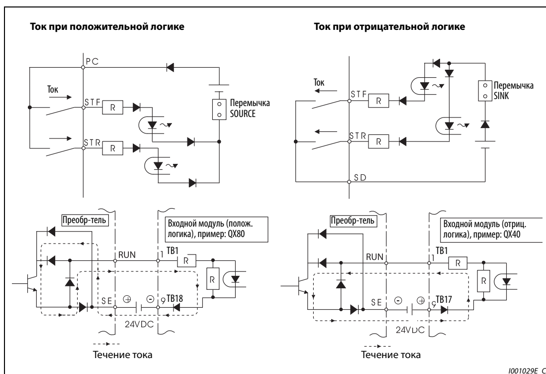
Рис. 2-27: Выбор управляющей логики
