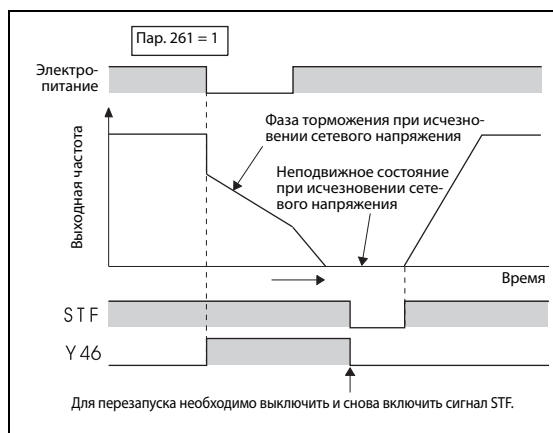
Рис. 5-215: Восстановление питания
