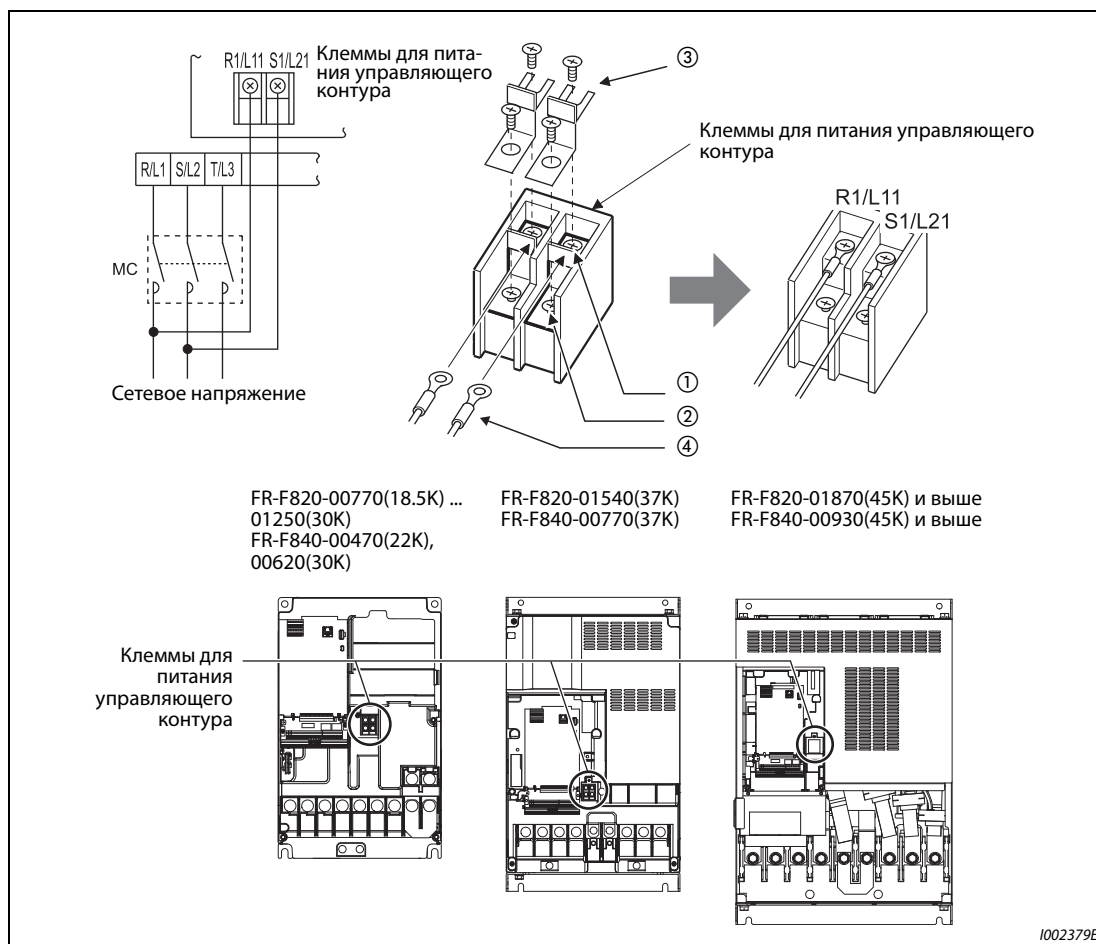
Рис. 2-42: Детальный вид клемм
