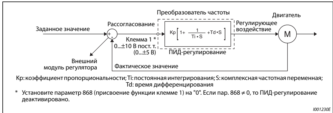
Рис. 5-159: Конфигурация системы для пар. 128 = 10, 11 (использование внешнего компаратора)
