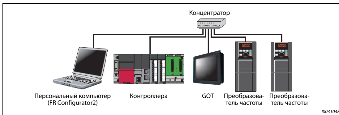
Рис. 2-59: Конфигурация системы для коммуникации по Ethernet
