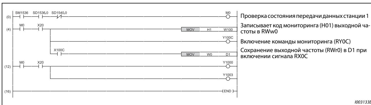
Рис. 5-293: Пример программы 4
