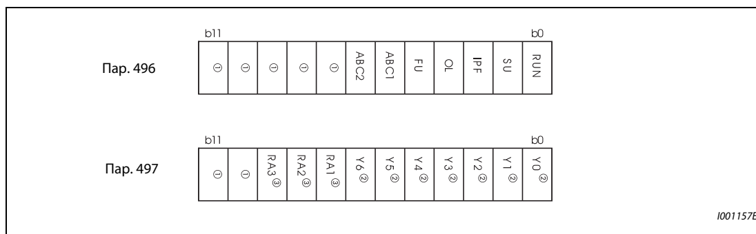
Рис. 5-104: Данные удаленного вывода
