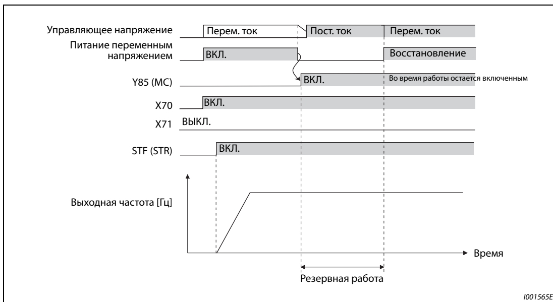
Рис. 5-275: Пример 3 работы при исчезновении сетевого напряжения (при непрерывной работе)
