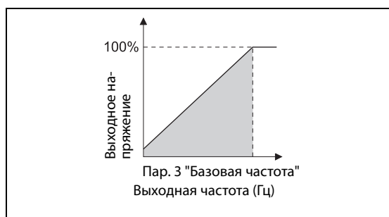
Рис. 5-261: Линейная характеристика
