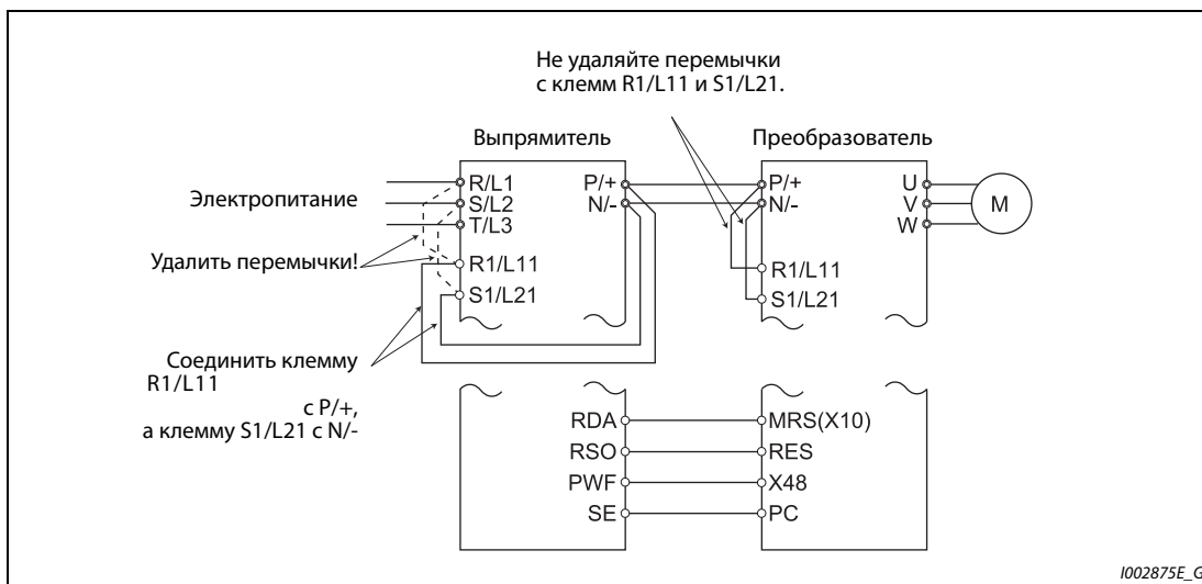
Рис. 5-213: Подключение преобразователя частоты с отдельным выпрямителем
