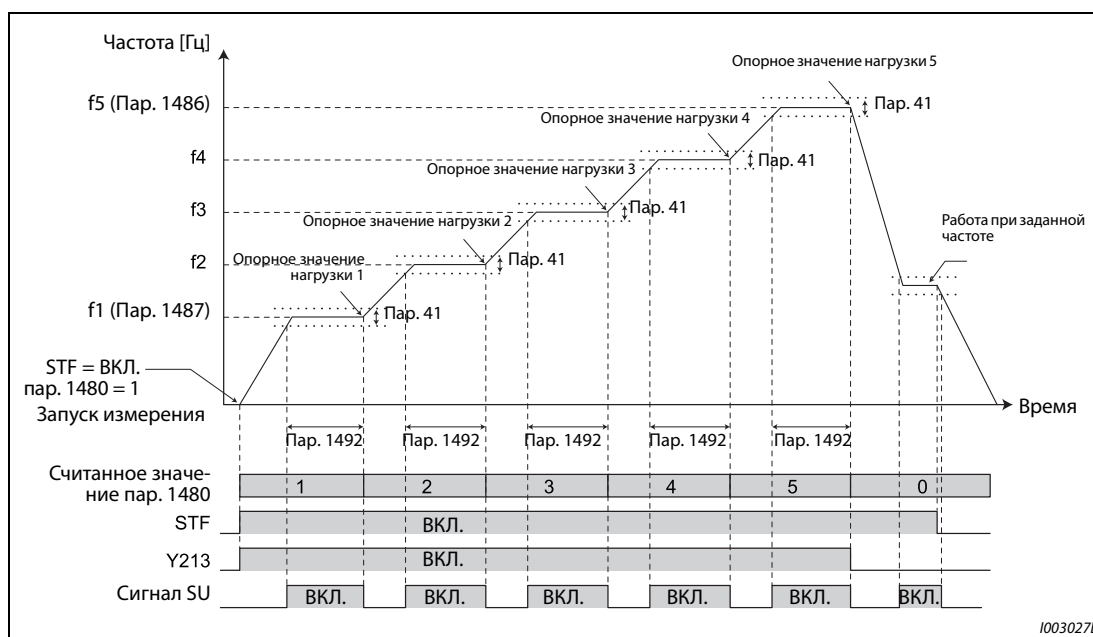
Рис. 5-72: Пример для запуска измерения из неподвижного состояния
