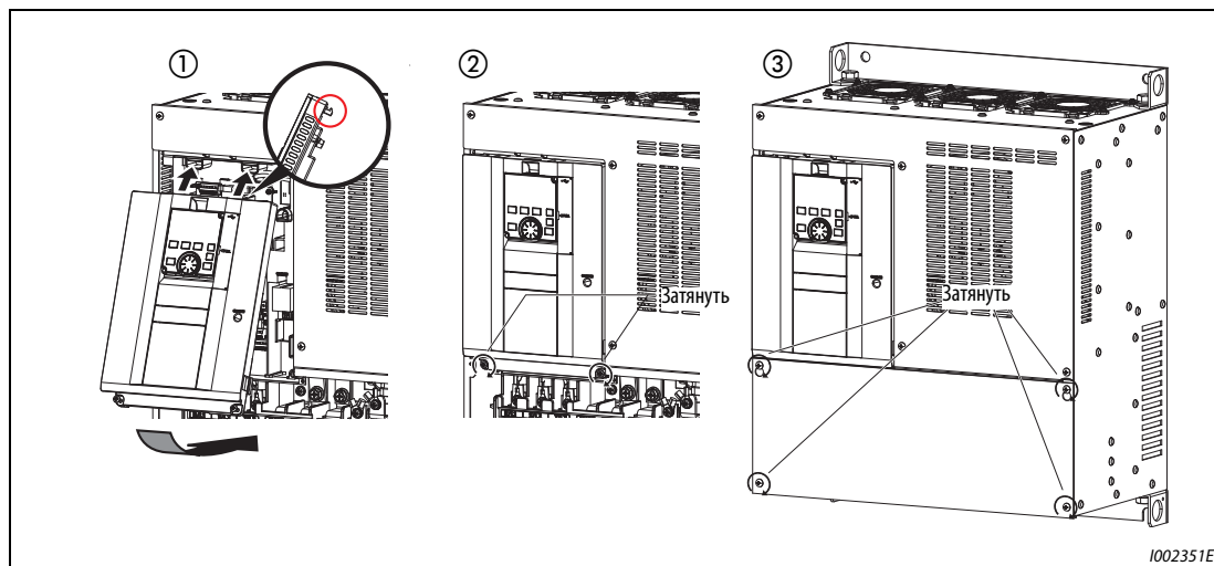
Рис. 2-12: Установка передних панелей
