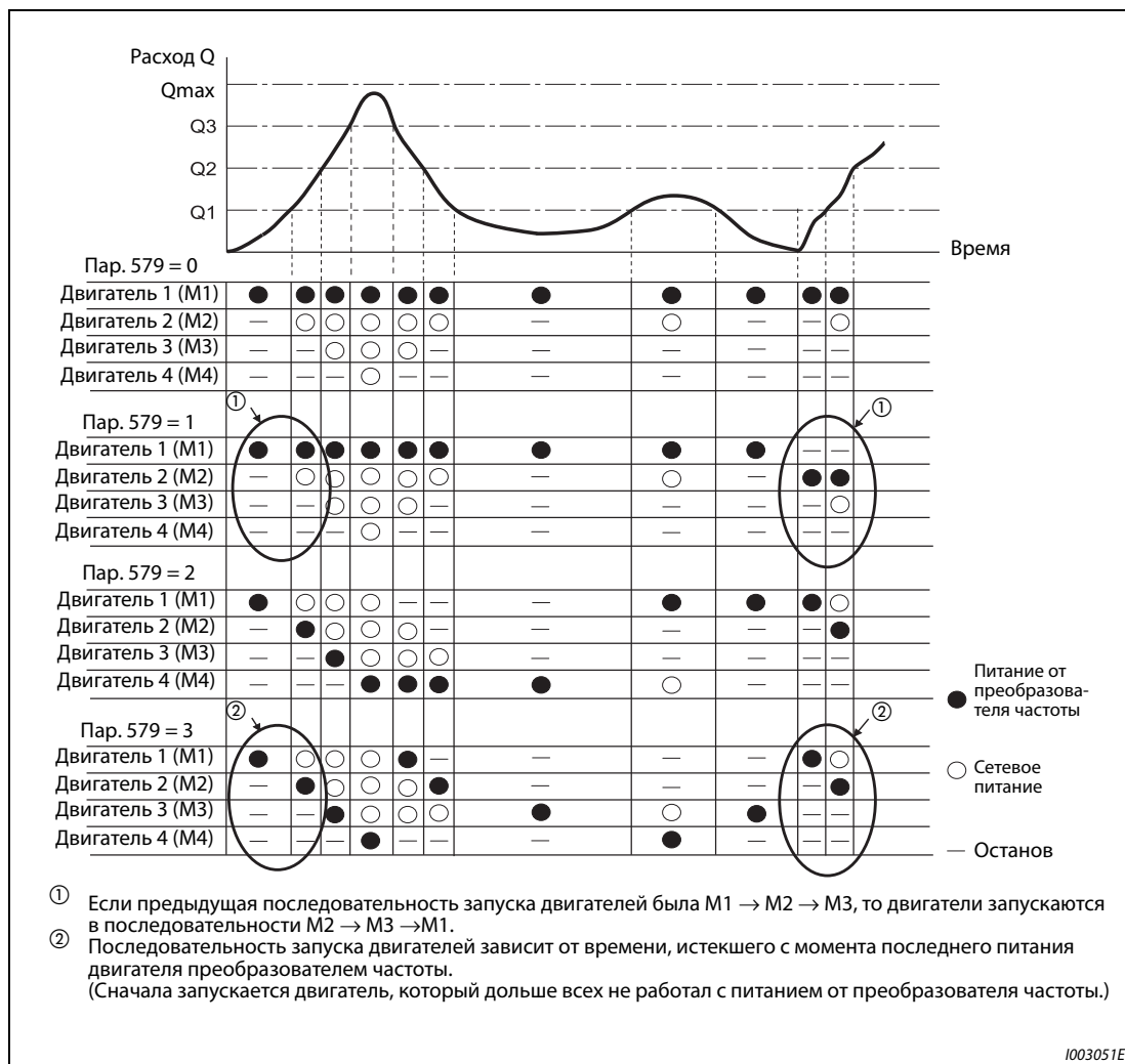
Рис. 5-185: Регулирование расхода жидкости через вспомогательные двигатели
