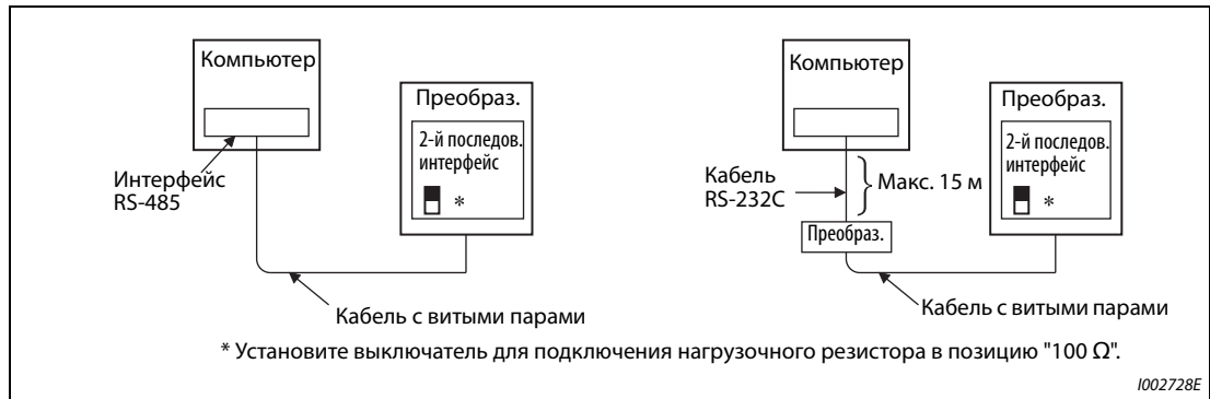
Рис. 5-226: Соединение с одним преобразователем частоты
