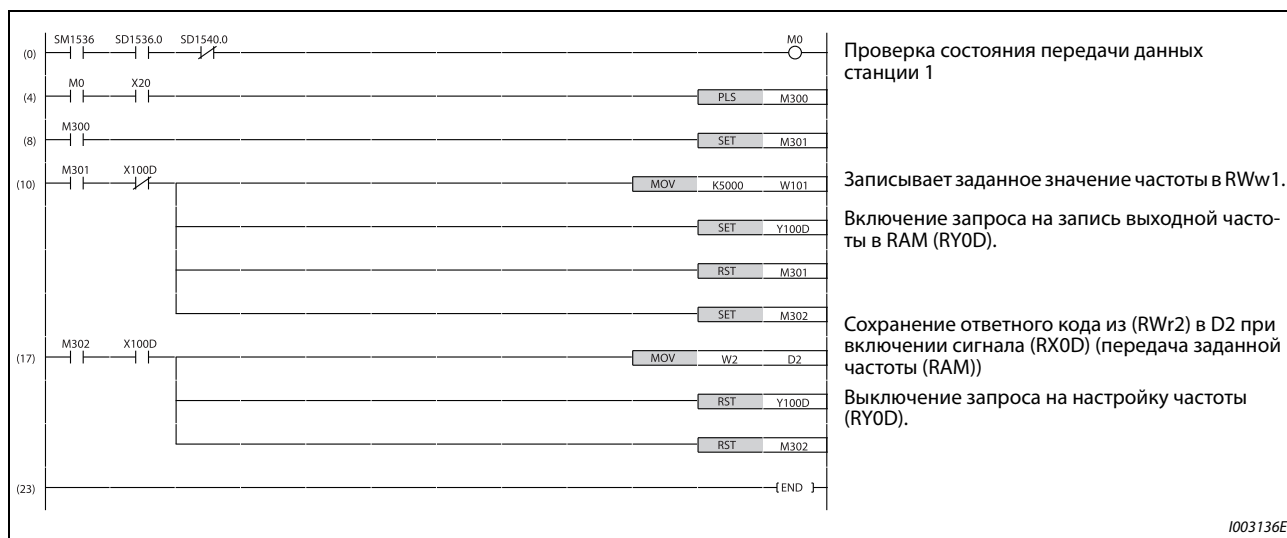
Рис. 5-296: Пример программы 7
