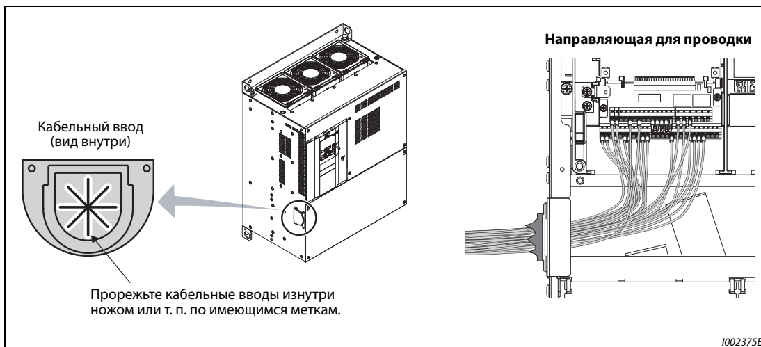
Рис. 2-38: Проводка управляющих сигналов моделей FR-F820-03160(75K) и выше, FR-F840-02160(90K) и выше
