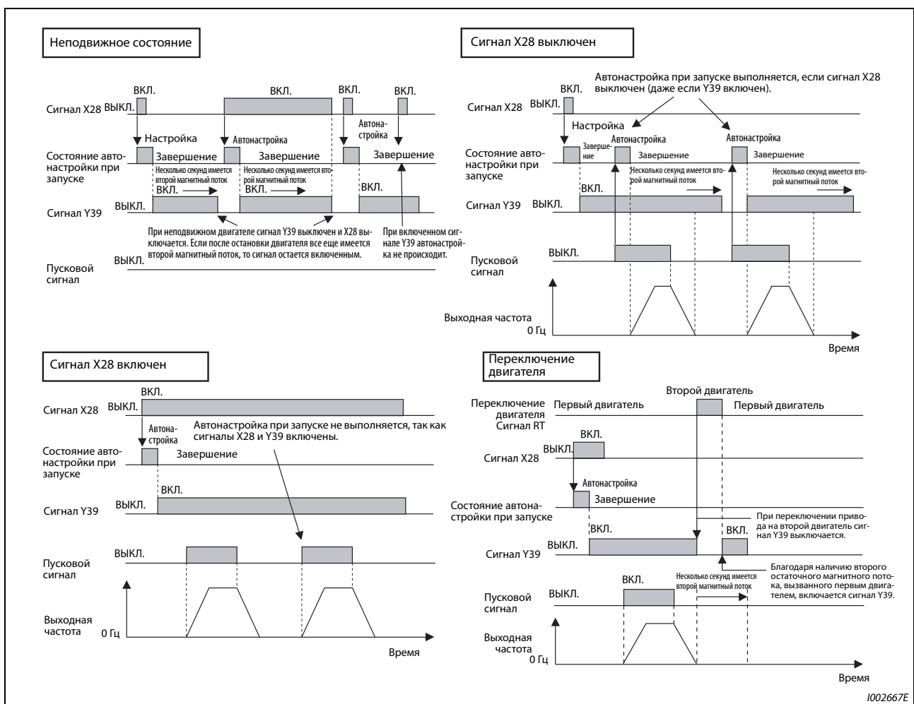
Рис. 5-144: Временные диаграммы онлайн-автонастройки параметров двигателя
