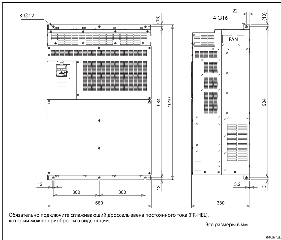
Рис. 8-11: Габаритно-присоединительные размеры преобразователей частоты FR-F840-05470(250K), 06100(280K), 06830(315K)
