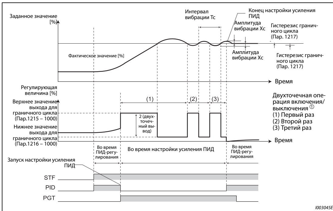
Рис. 5-176: Пример временной последовательности
