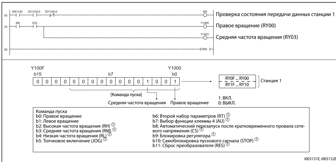
Рис. 5-292: Пример программы 3
