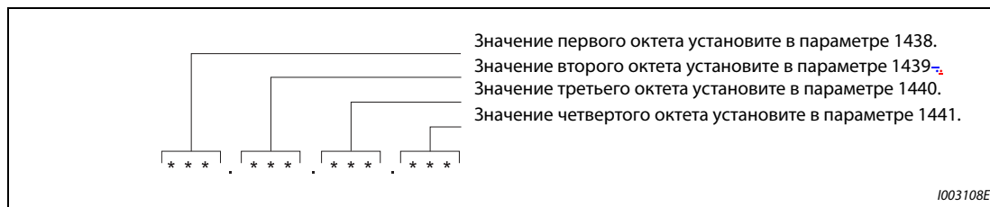
Рис. 5-249: Настройка маски подсети
