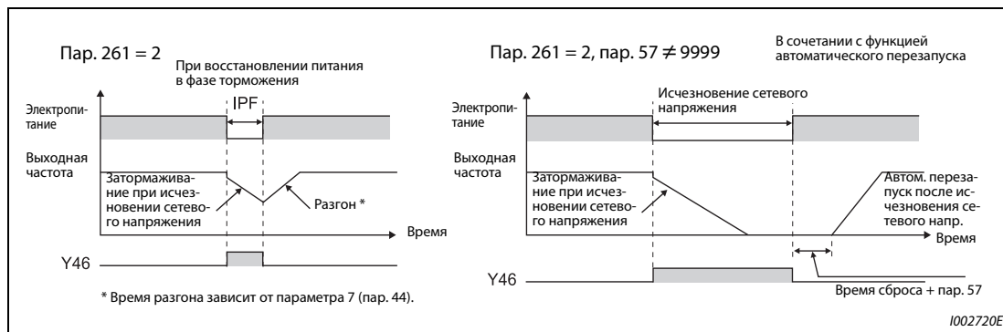
Рис. 5-216: Продолжение работы после исчезновения сетевого напряжения
