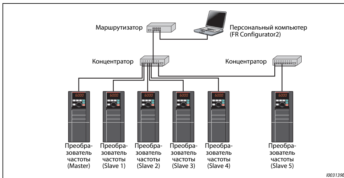
Рис. 5-299: Конфигурация системы для функции связи "преобразователь с преобразователем".
