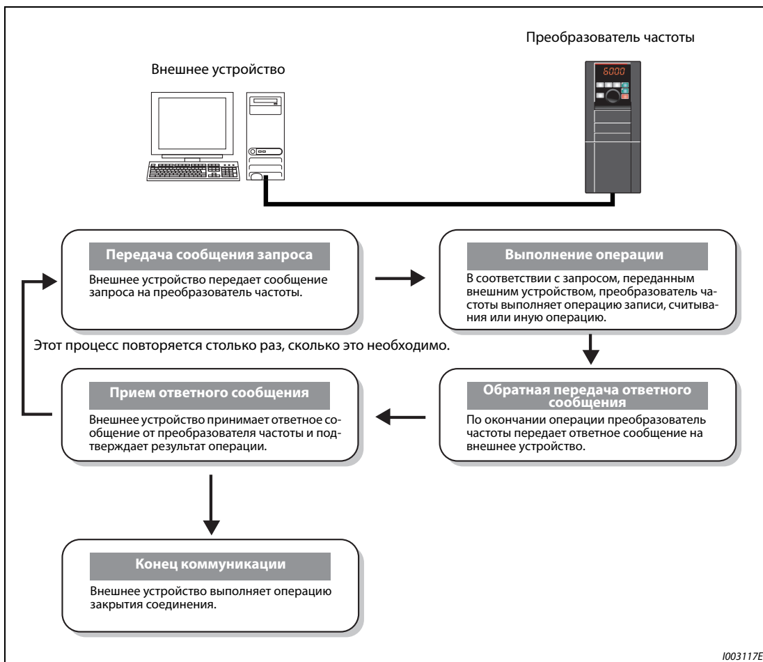
Рис. 5-282: Процесс коммуникации по протоколу UDP/IP
