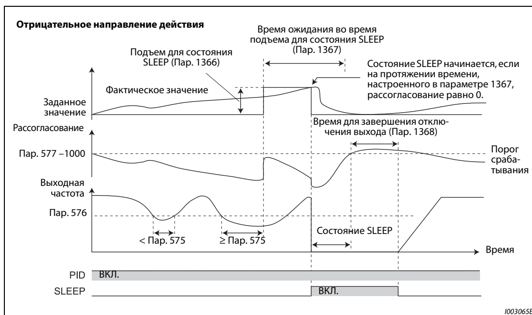
Рис. 5-199: Подъем ПИД при SLEEP
