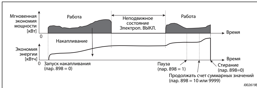
Рис. 5-92: Накопление экономии энергии
