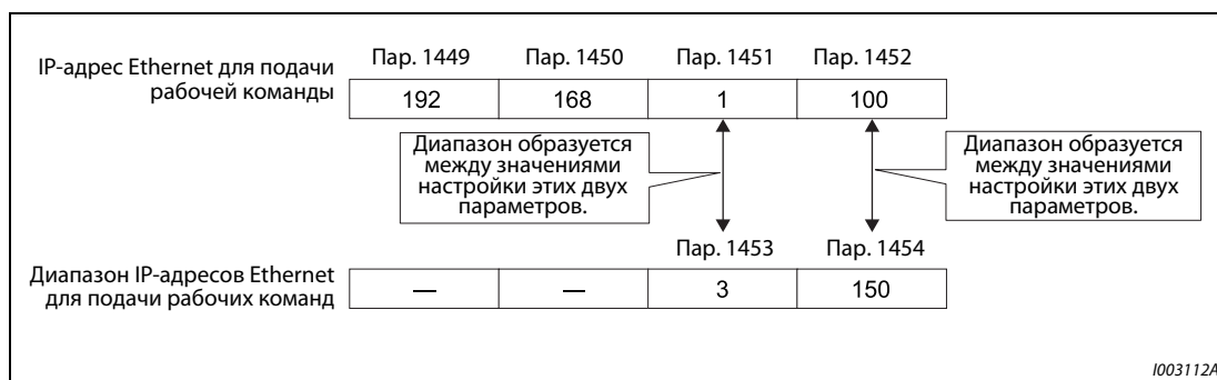
Рис. 5-253: Пример 1 настройки диапазона IP-адресов для подачи рабочих команд
