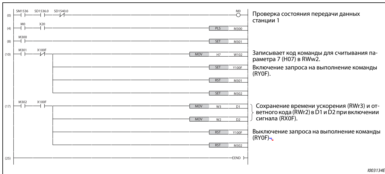
Рис. 5-294: Пример программы 5
