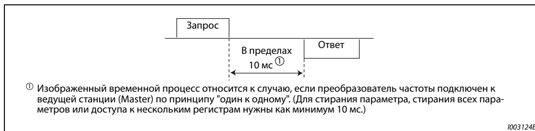
Рис. 5-285: Формат сообщений
