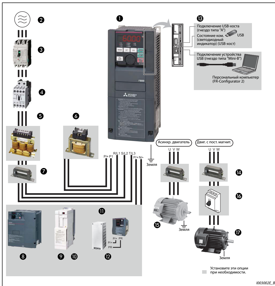
Рис. 2-1: Обзор конфигурации системы
