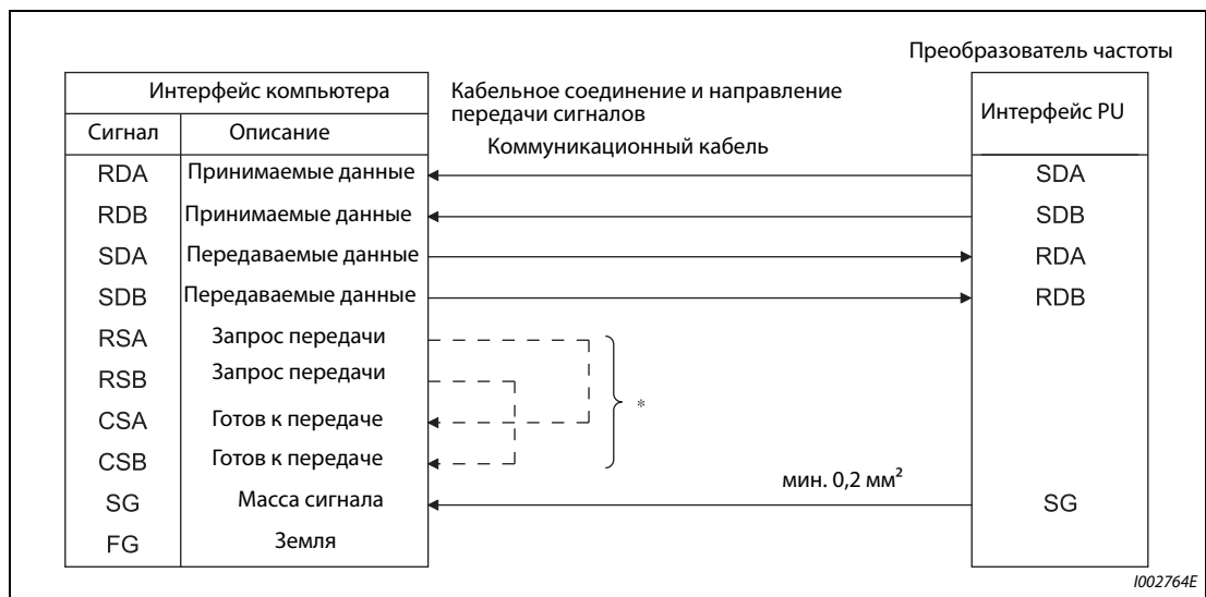
Рис. 5-224: Соединение с одним преобразователем частоты
