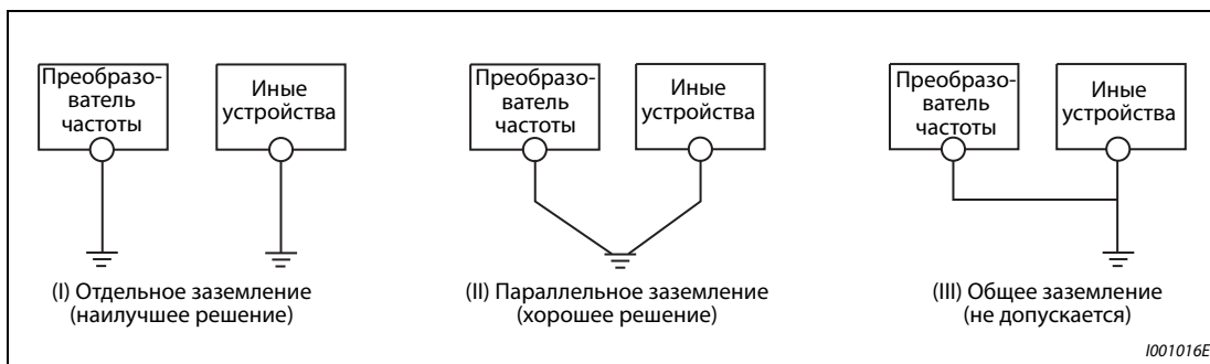
Рис. 2-25: Заземление системы привода
