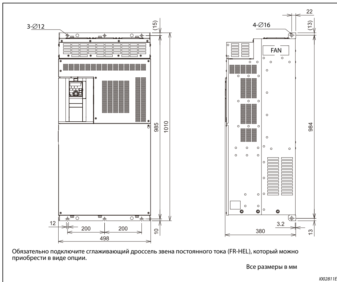
Рис. 8-10: Габаритно-присоединительные размеры преобразователей частоты FR-F840-04320(185K), 04810(220K)
