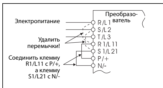
Рис. 5-212: Подключение стандартной модели
