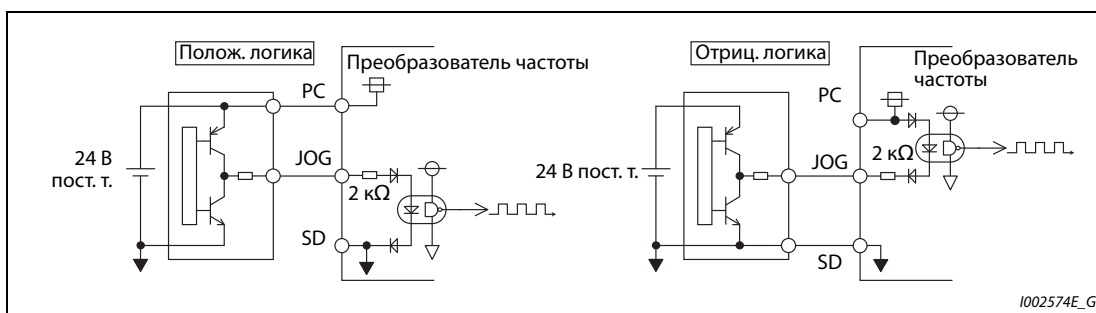
Рис. 5-38: Импульсный выход
