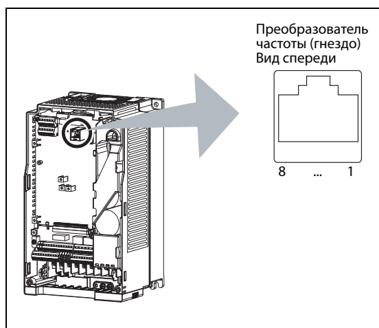
Рис. 5-222: Разводка контактов разъема PU
