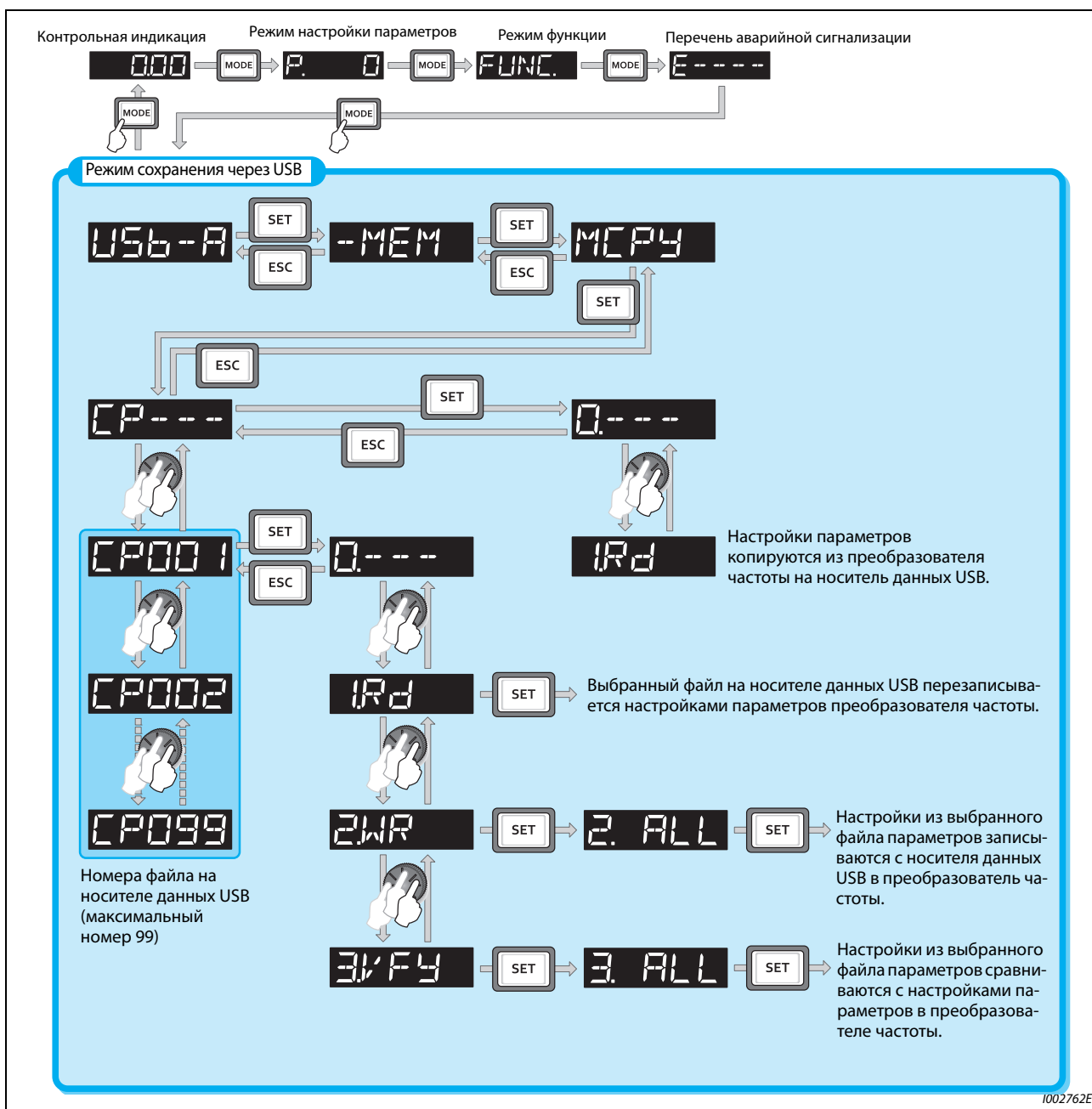
Рис. 5-280: Функции в режиме сохранения через USB
