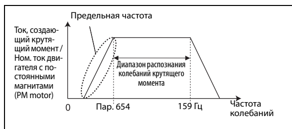
Рис. 5-279: Настройка
