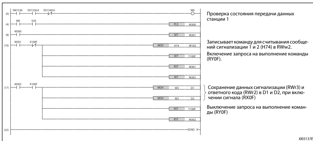
Рис. 5-297: Пример программы 8
