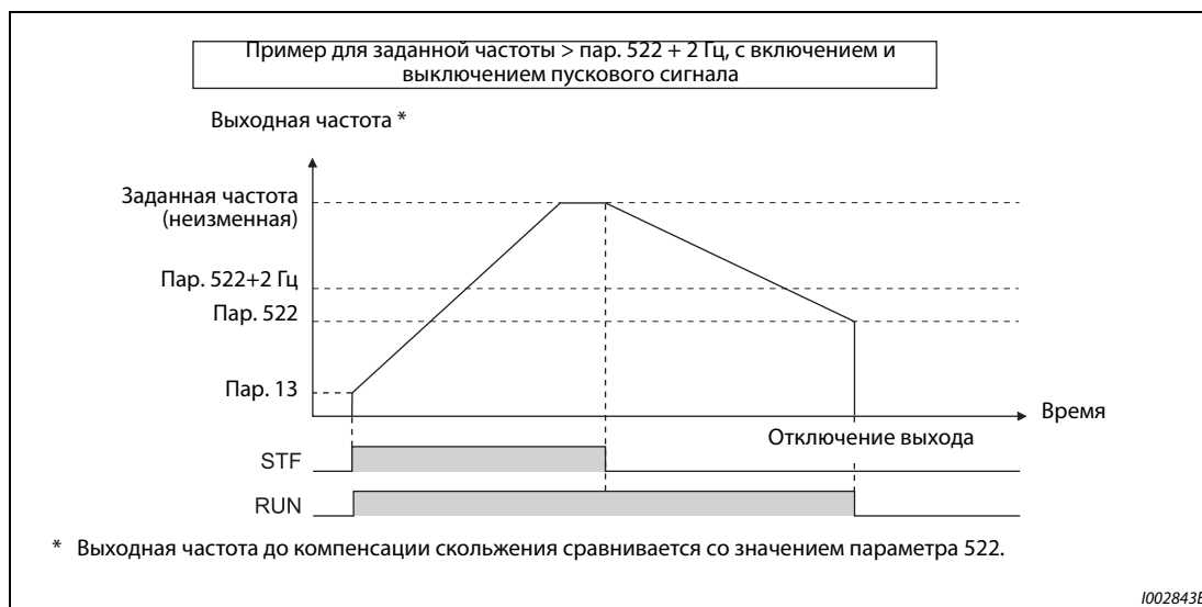
Рис. 5-266: Пример отключения выхода
