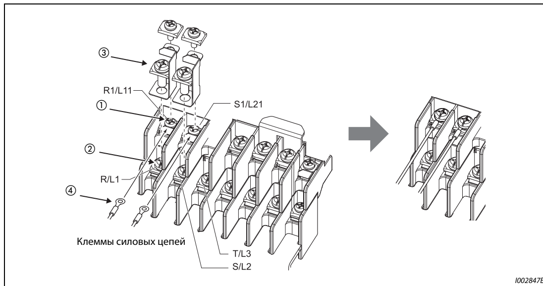
Рис. 2-41: Детальный вид клемм
