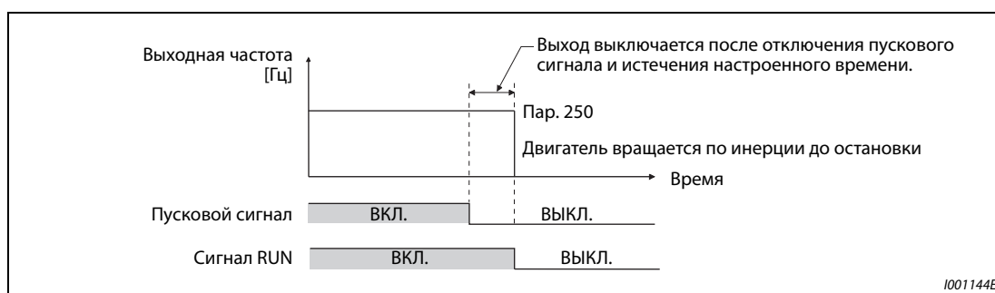
Рис. 5-269: Метод останова при пар. 250 ≠ 8888 и 9999
