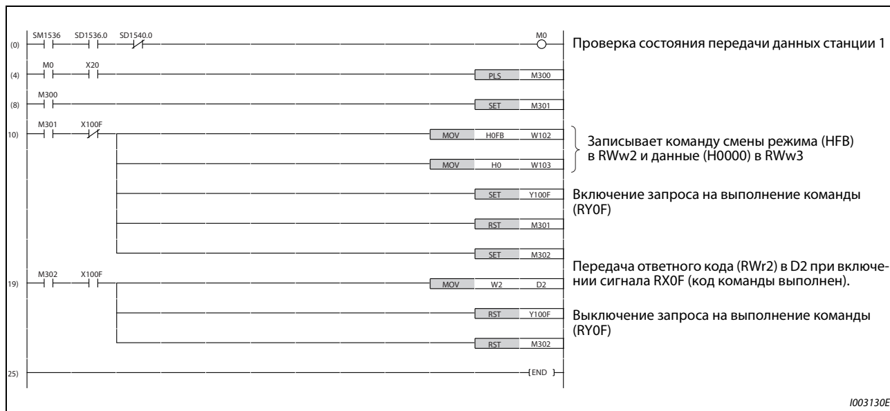
Рис. 5-291: Пример программы 2
