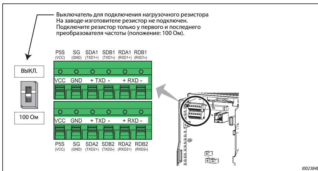
Рис. 2-47: 2-й последовательный интерфейс преобразователя частоты
