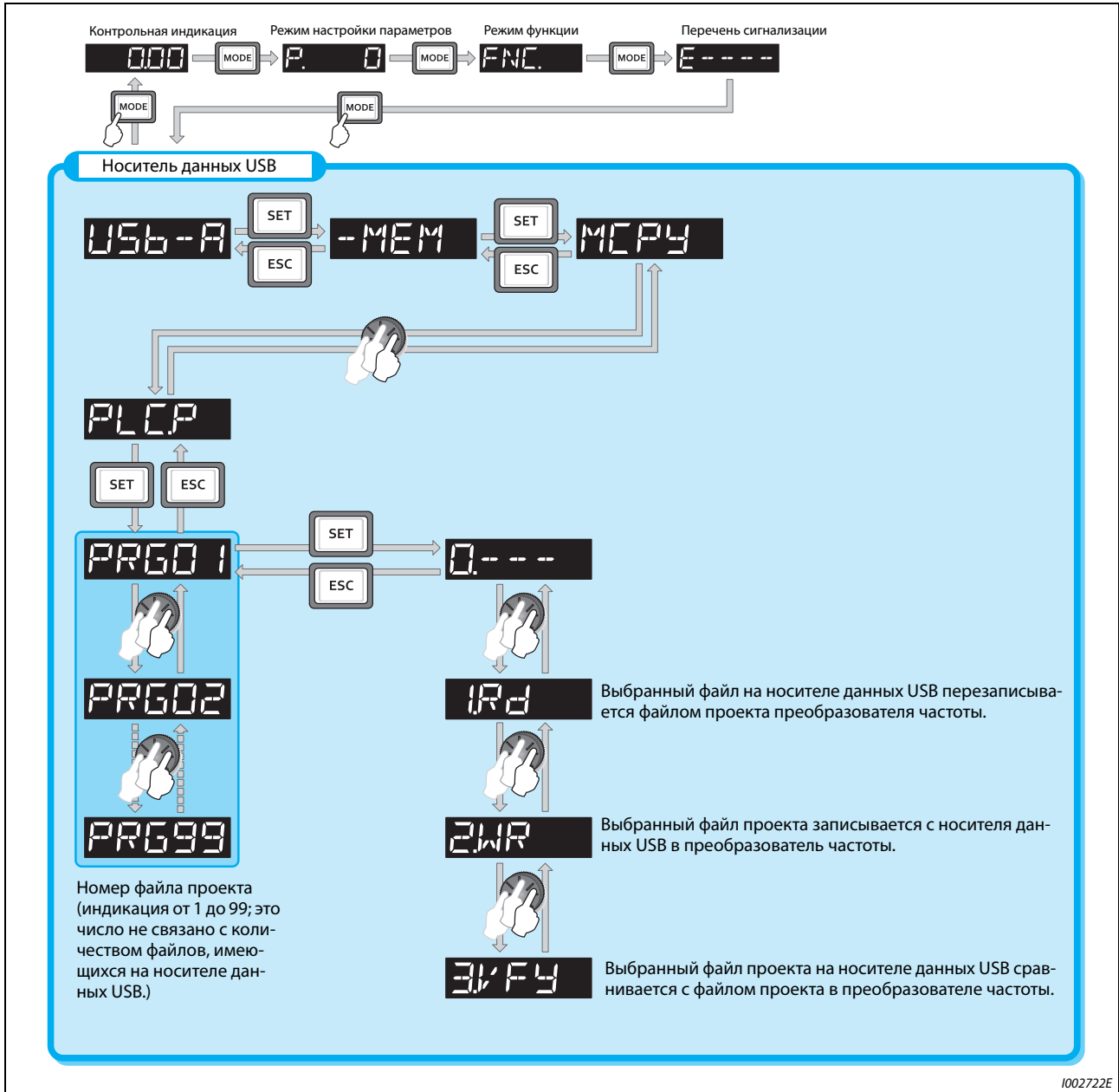
Рис. 5-218: Копирование проектных данных функции контроллера на носитель данных USB
