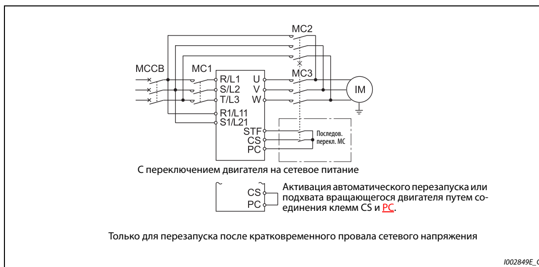
Рис. 5-205: Пример подключения
