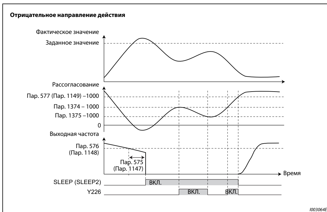
Рис. 5-198: ПИД-функция дополнительного нагнетательного насоса
