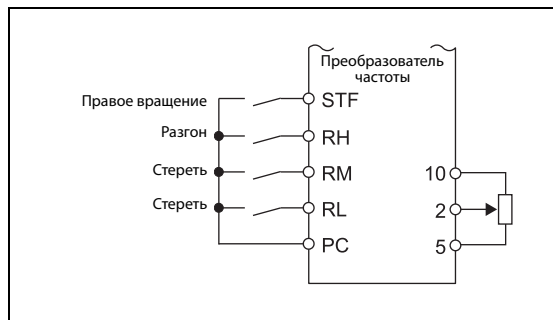
Рис. 5-25: Пример схемы для использования цифрового потенциометра
