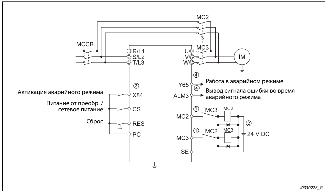
Рис. 5-58: Внешнее подключение выводов для аварийного режима
