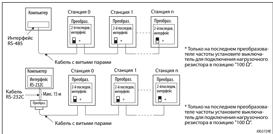
Рис. 5-227: Соединение с несколькими преобразователями частоты
