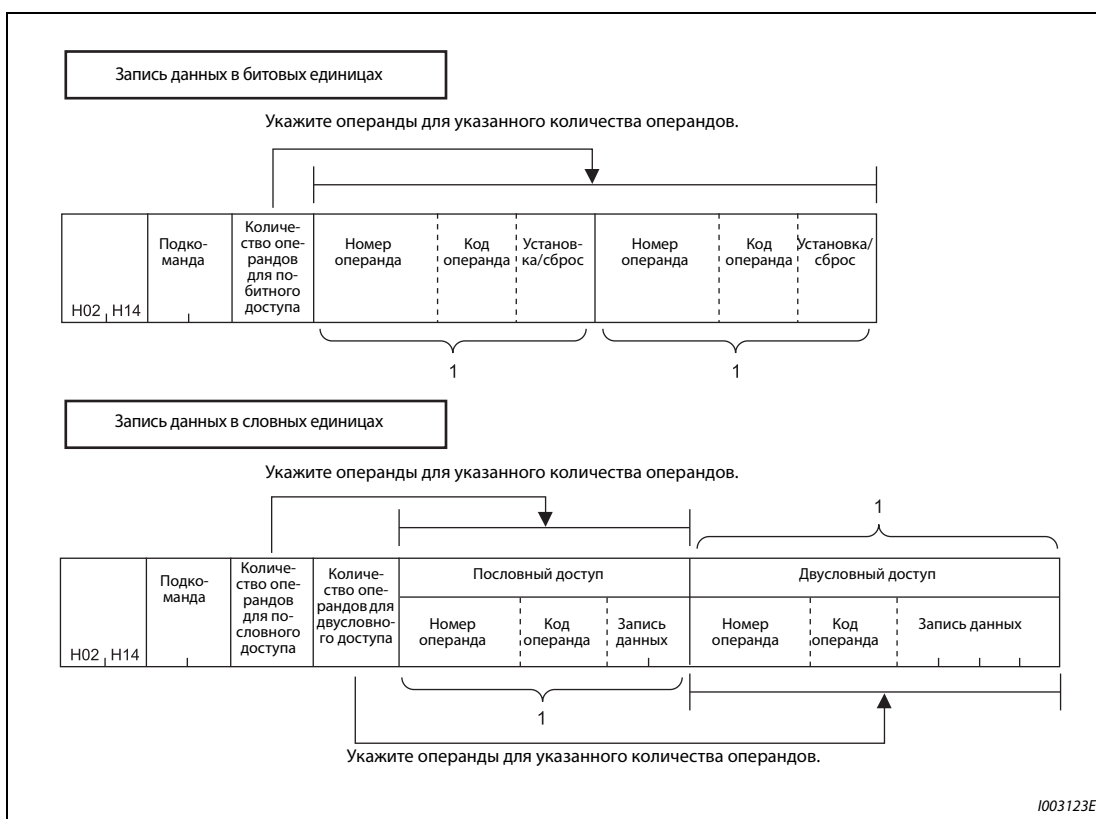
Рис. 5-284: Данные запроса для произвольной записи
