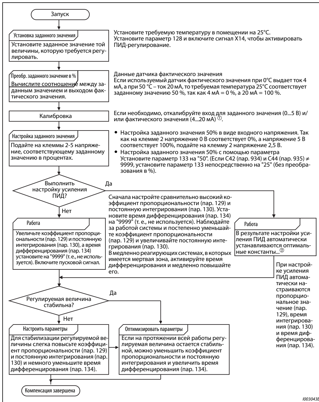
Рис. 5-173: Пример компенсации
