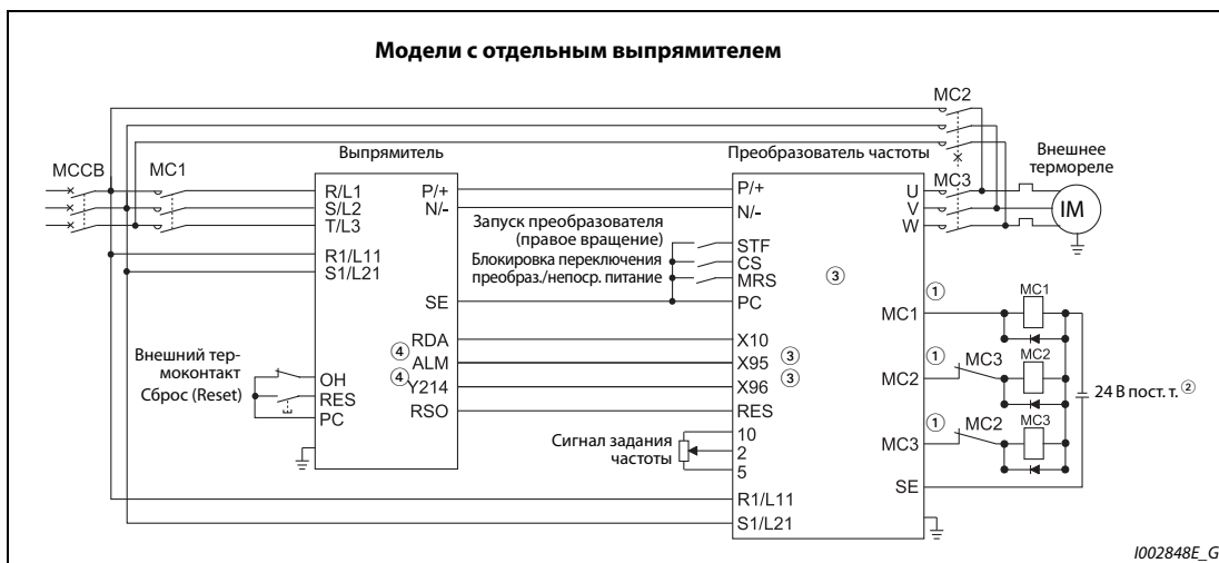
Рис. 5-146: Подключение силовых контакторов (модели с отдельным выпрямителем)
