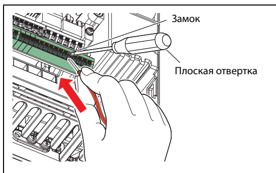
Рис. 2-34: Подсоединение многопроволочного провода
