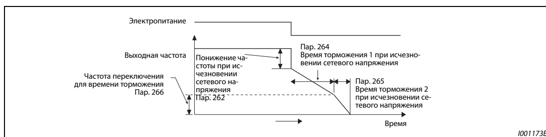
Рис. 5-214: Параметры метода останова при исчезновении сетевого напряжения
