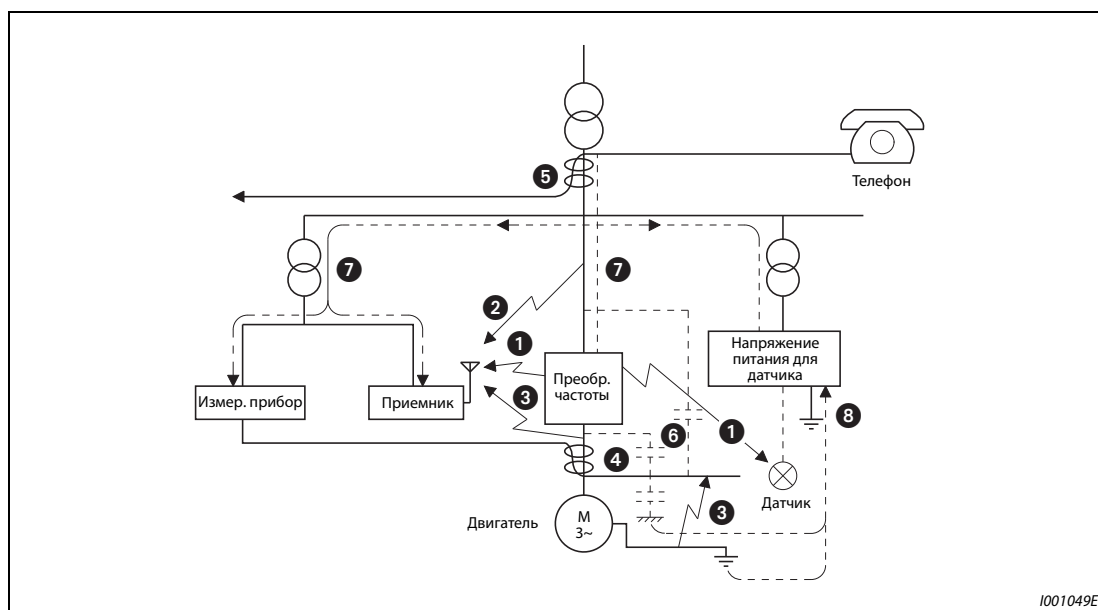
Рис. 3-4: Пути распространения помех
