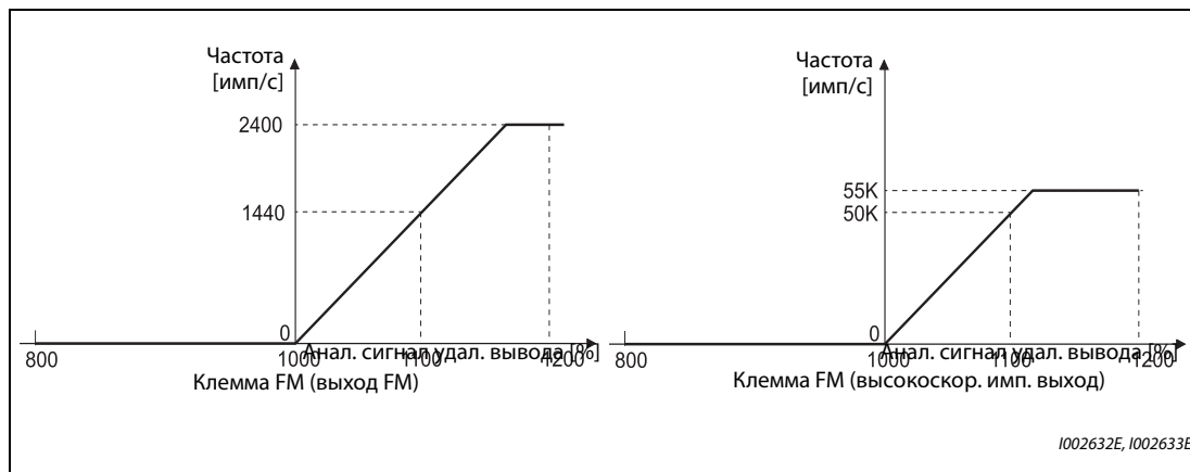
Рис. 5-106: Вывод через клемму FM
