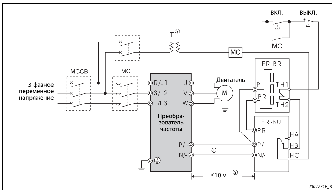
Рис. 2-51: Подключение тормозного блока FR-BU
