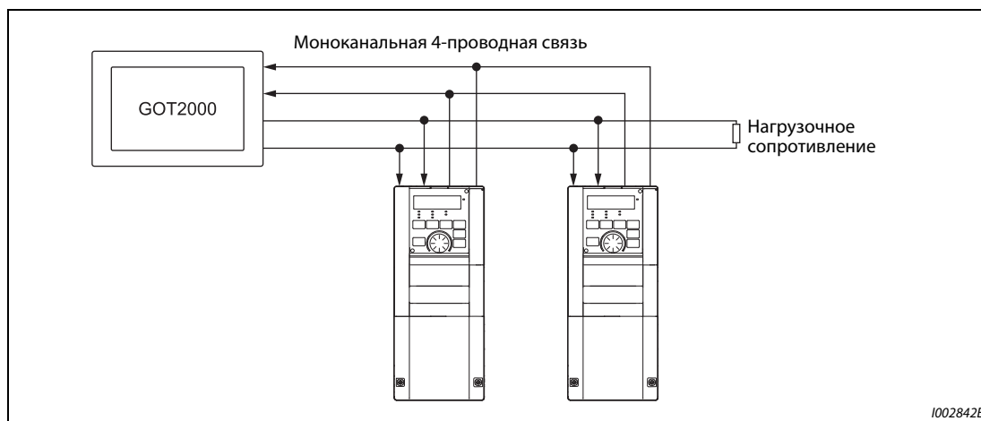
Рис. 5-258: Автоматическая связь с GOT2000
