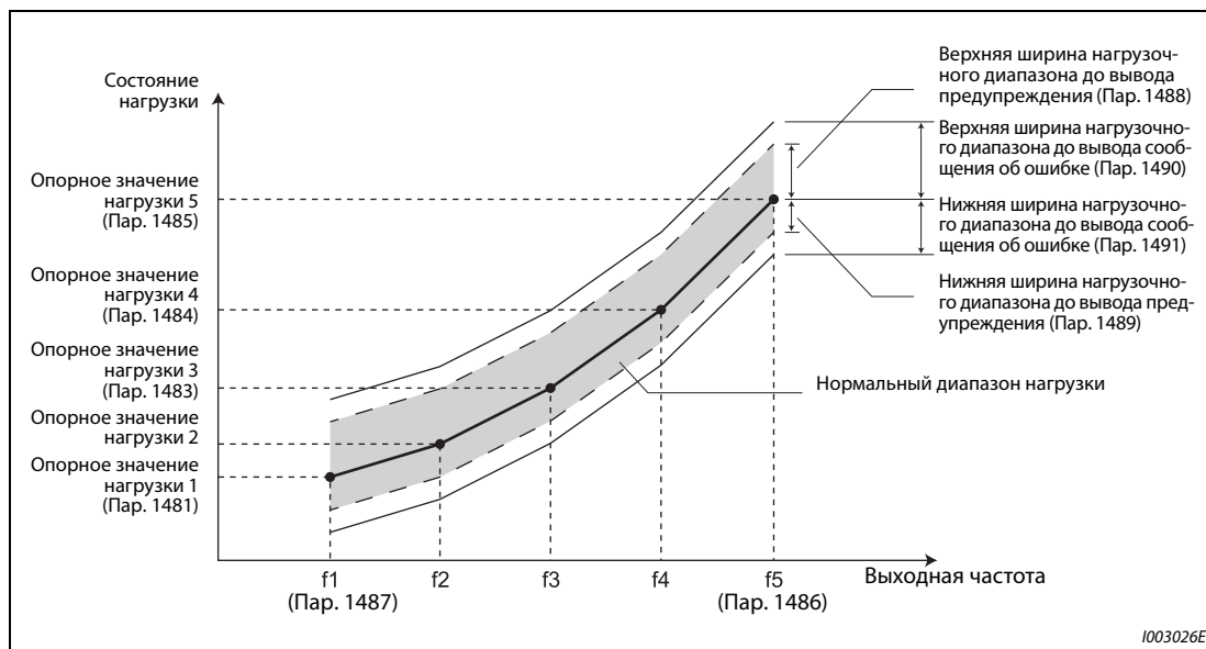
Рис. 5-71: Настройка нагрузочной характеристики и диапазона выходной частоты
