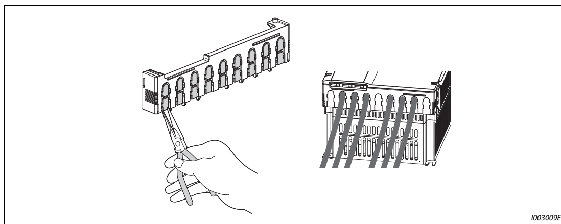
Рис. 2-23: Гребенка для ввода кабелей
