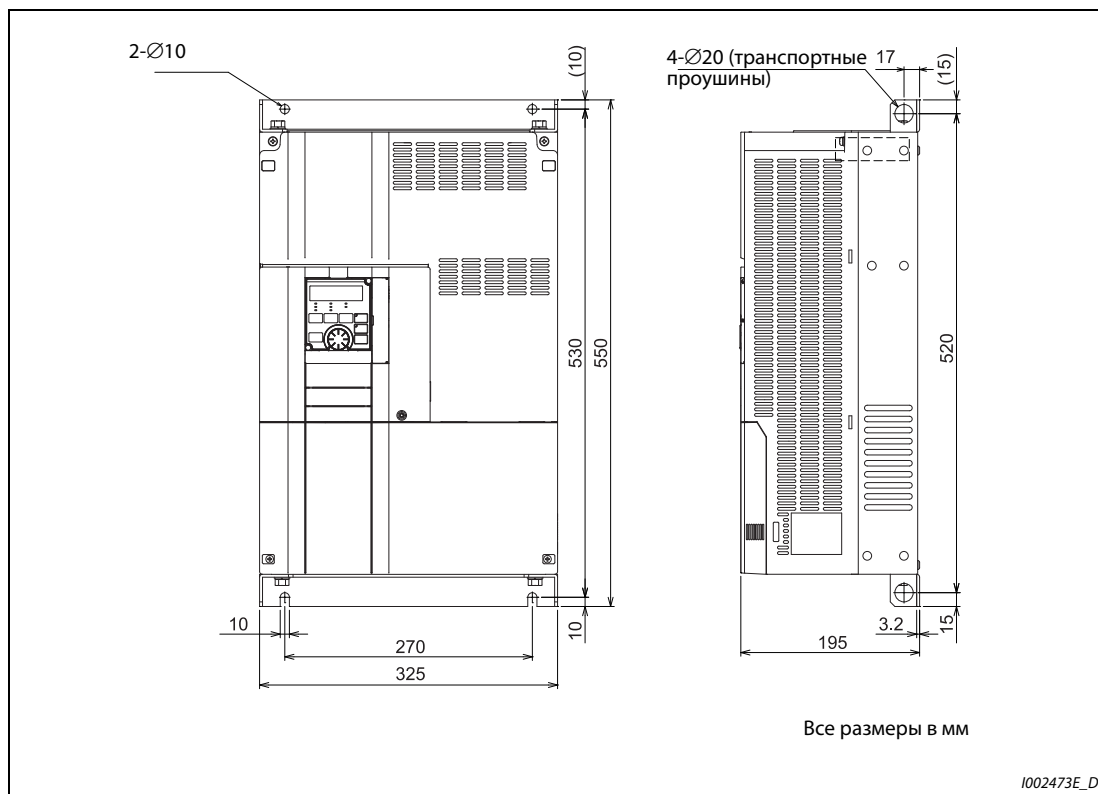
Рис. 8-8: Габаритно-присоединительные размеры преобразователей частоты FR-F820-01540(37K), FR-F840-00770(37K)
