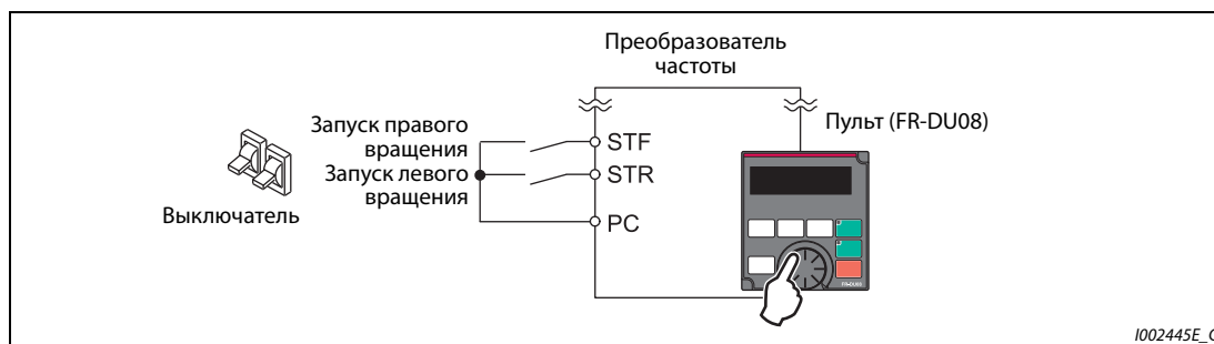
Рис. 4-8: Внешнее управление
