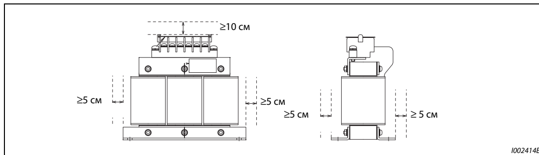
Рис. 2-56: Минимальные расстояния для дросселя звена постоянного тока (FR-HEL)
