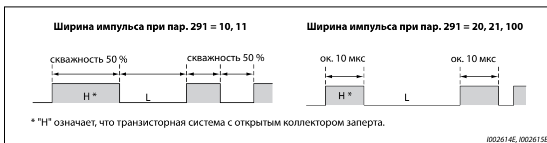
Рис. 5-87: Две различные ширины импульсов
