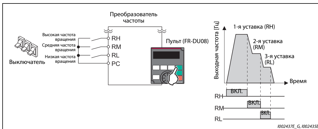
Рис. 4-5: Вызов уставки частоты вращения (скорости) с помощью выключателя
