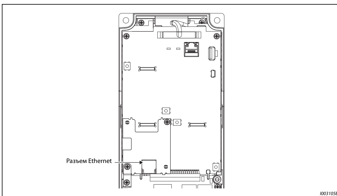
Рис. 2-60: Местоположение порта Ethernet
