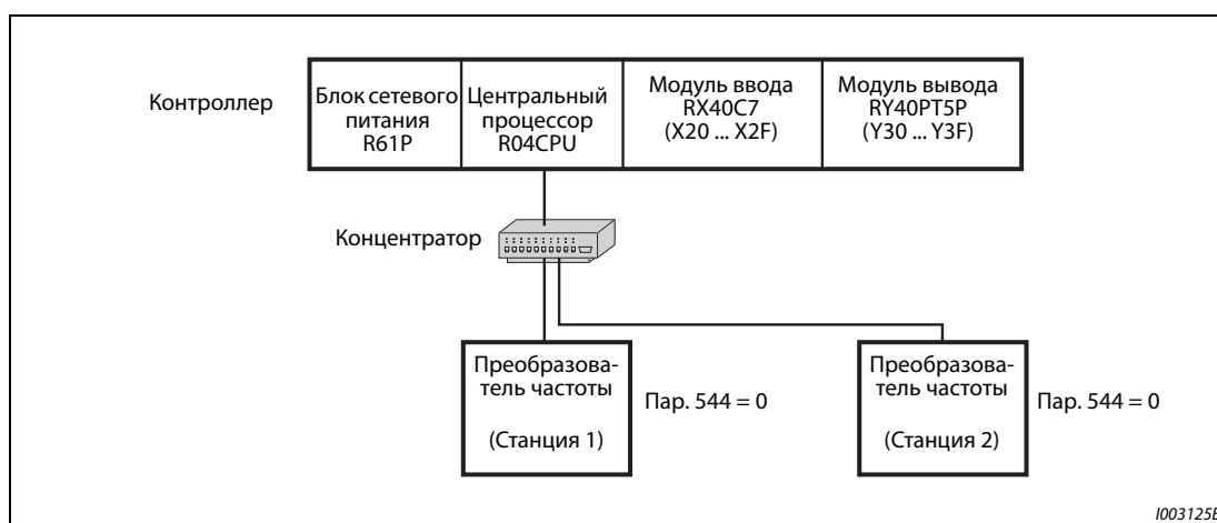
Рис. 5-287: Сеть CC-Link IEF Basic с контроллером и двумя преобразователями частоты
