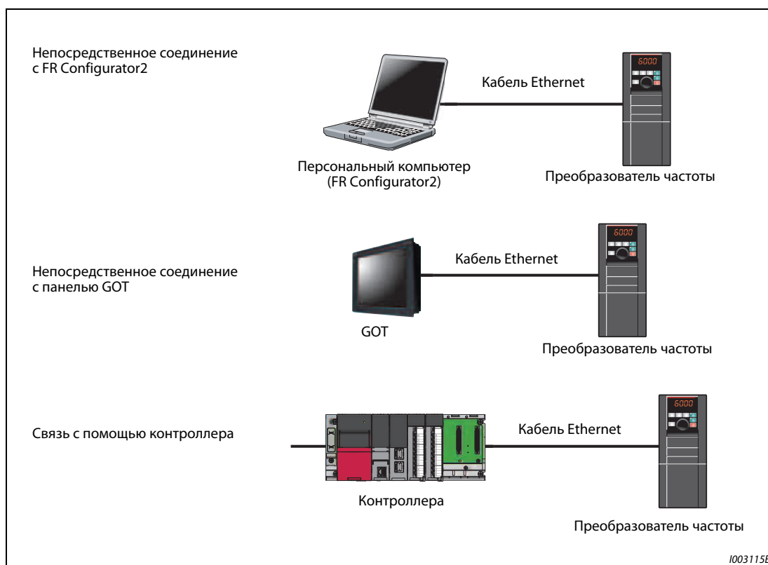
Рис. 5-256: Конфигурация привязки к продукции MELSOFT / FA
