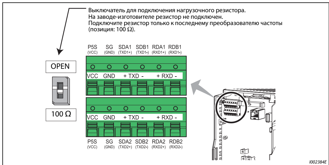
Рис. 5-225: 2-й последовательный интерфейс преобразователя частоты
