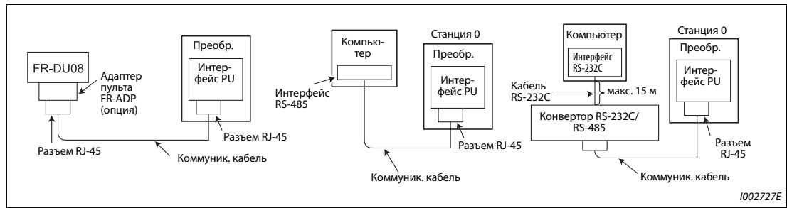
Рис. 5-223: Подключение интерфейса PU
