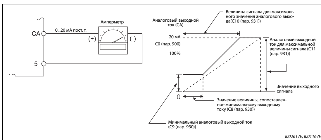
Рис. 5-89: Калибровка выхода CA
