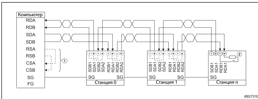
Рис. 5-229: Соединение с несколькими преобразователями частоты
