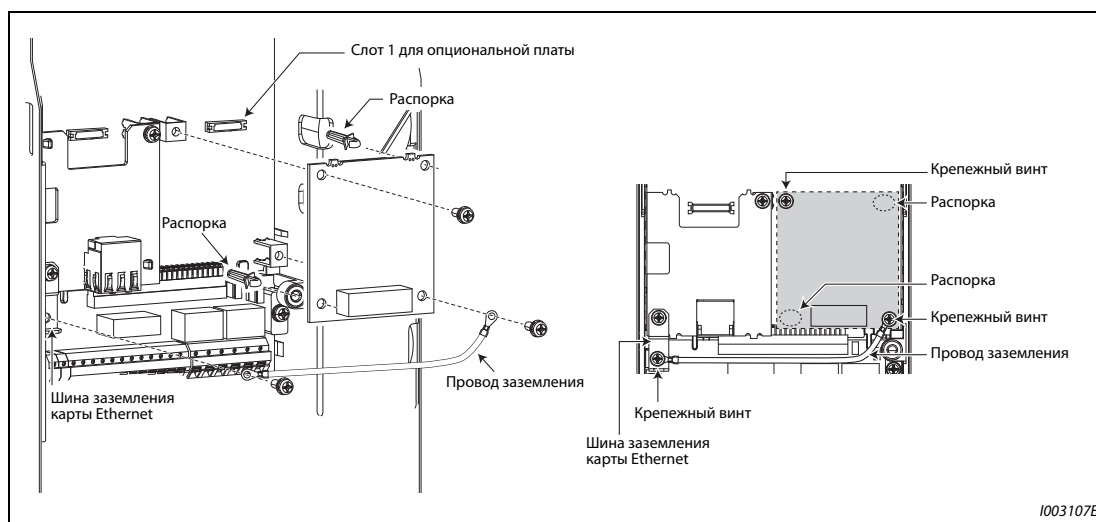
Рис. 2-58: Установка коммуникационной опции на FR-F800-E на примере карты FR-A8NC
