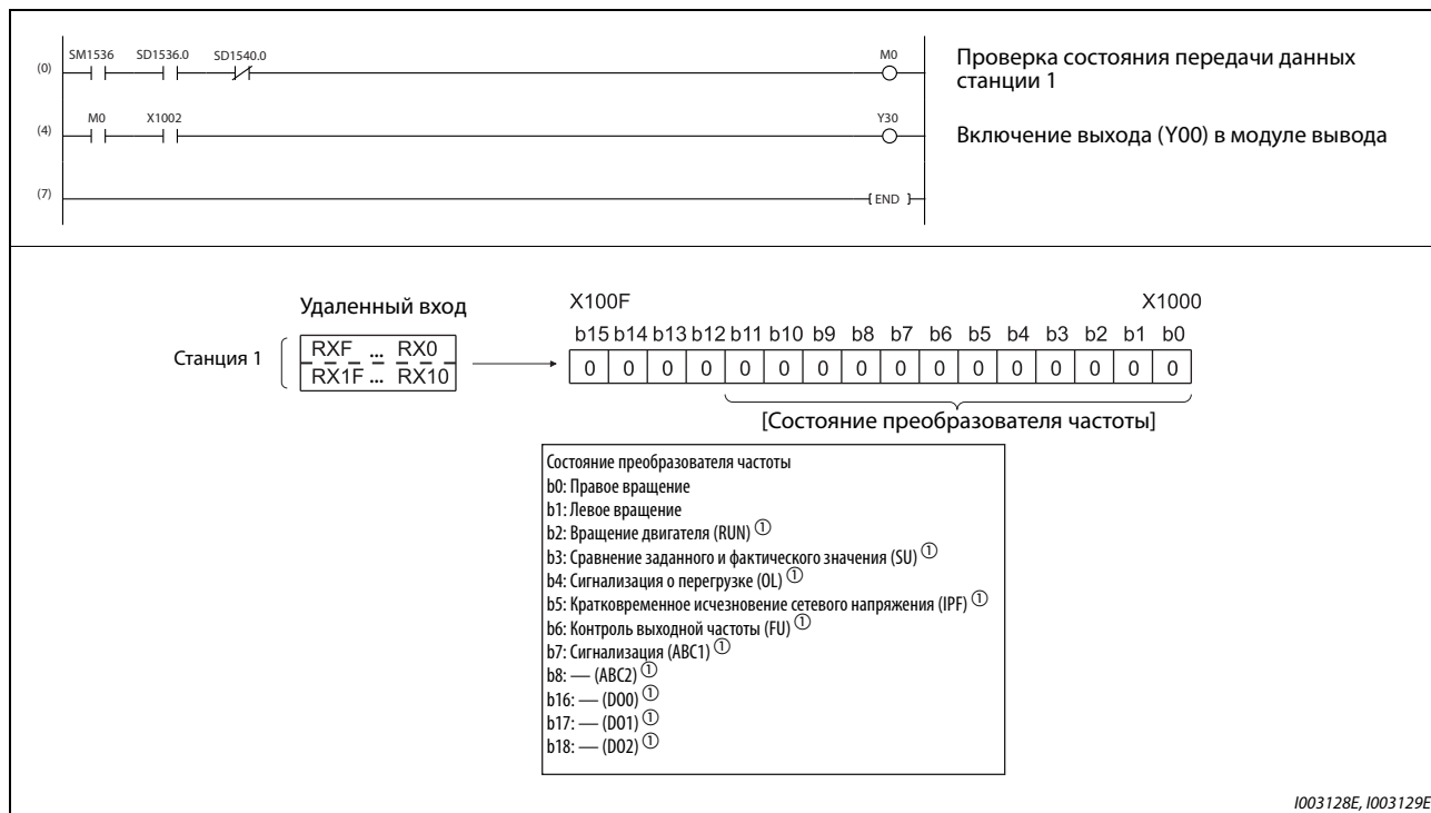
Рис. 5-290: Пример программы 1
