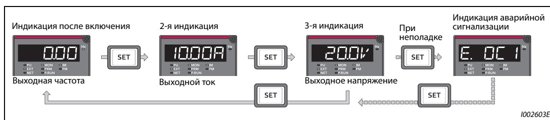
Рис. 5-76: Индикация различных рабочих величин
