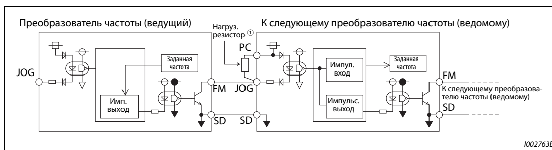
Рис. 5-40: Синхронизация частоты вращения (отрицательная схемная логика)
