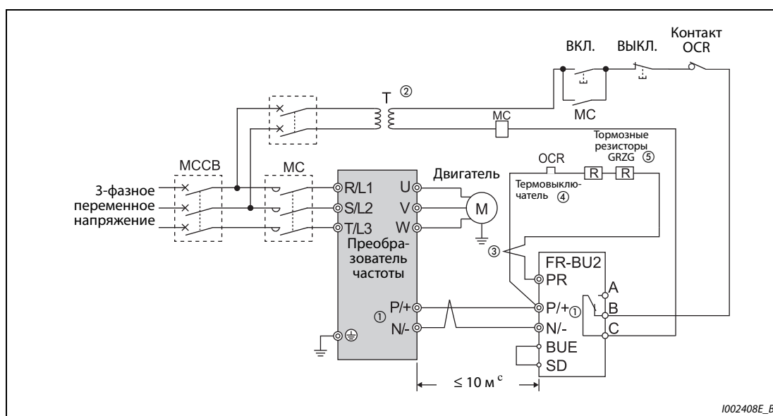
Рис. 2-48: Подключение тормозного блока с тормозным резистором GRZG
