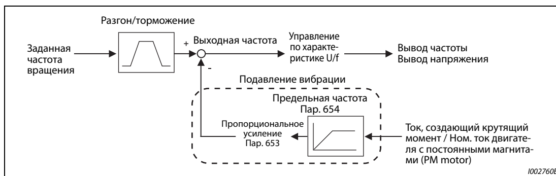
Рис. 5-278: Блок-схема
