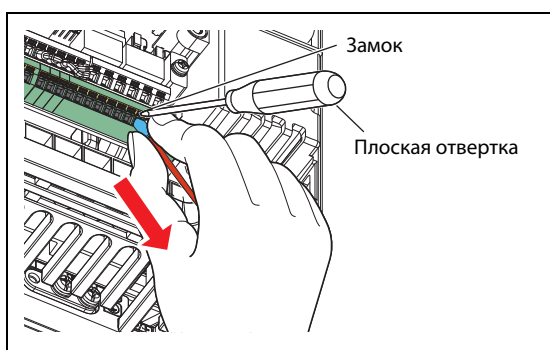
Рис. 2-35: Удаление провода
