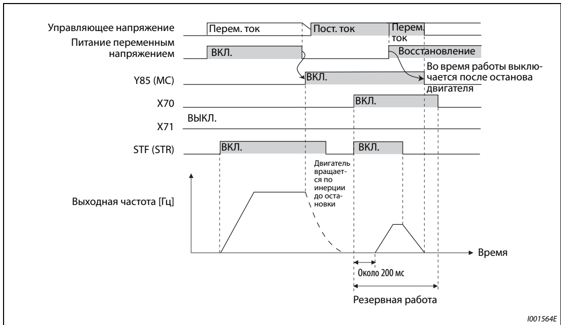
Рис. 5-274: Пример 2 работы при исчезновении сетевого напряжения (после восстановления напряжения питания)
