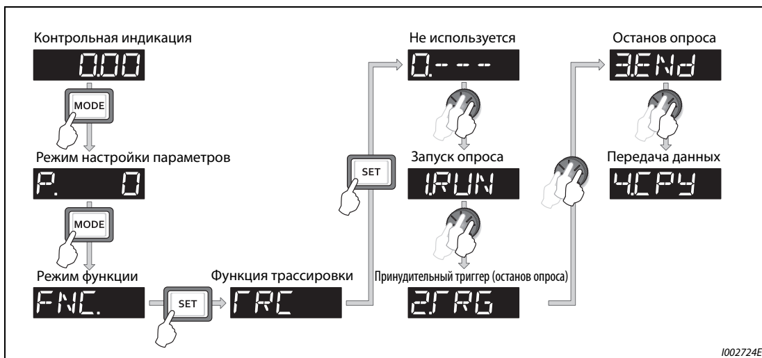
Рис. 5-220: Выбор функции трассировки
