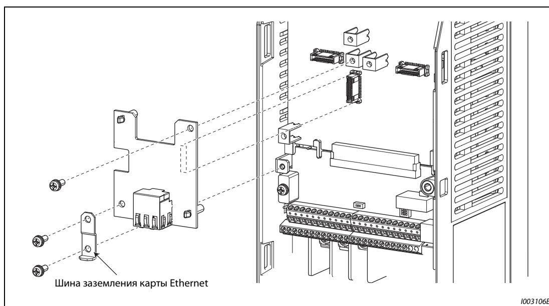
Рис. 2-61: Удаление карты Ethernet
