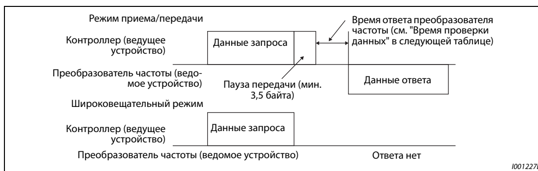
Рис. 5-242: Формат сообщений
