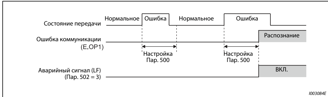
Рис. 5-233: Распознавание ошибки коммуникации в зависимости от настройки параметра 500
