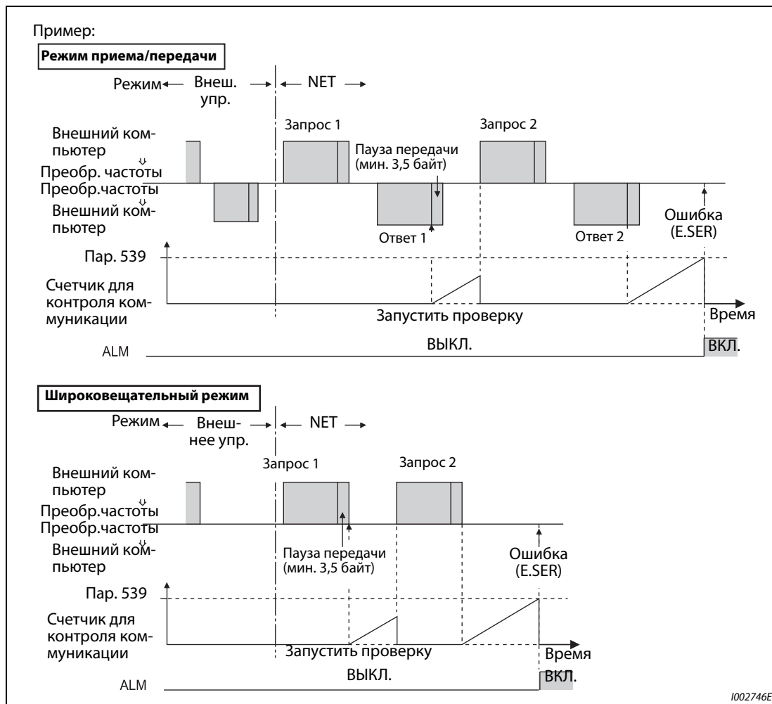
Рис. 5-245: Контроль на обрыв кабеля
