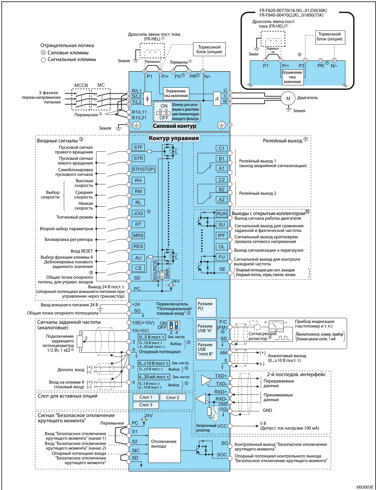
Рис. 2-20: Схема подключения преобразователя частоты (тип FM)
