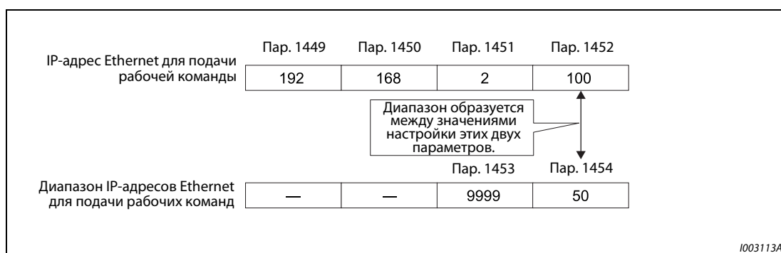
Рис. 5-254: Пример 2 настройки диапазона IP-адресов для подачи рабочих команд
