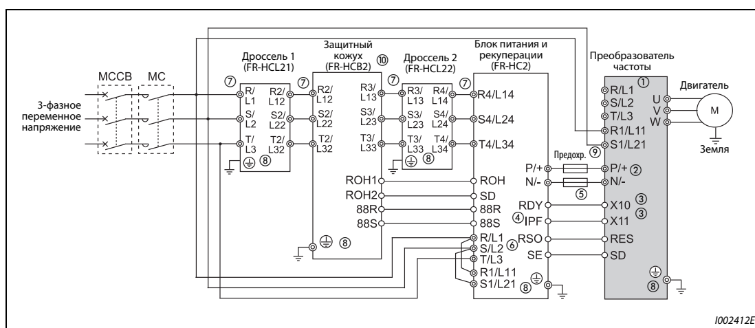
Рис. 2-53: Подключение блока питания и рекуперации FR-HC2
