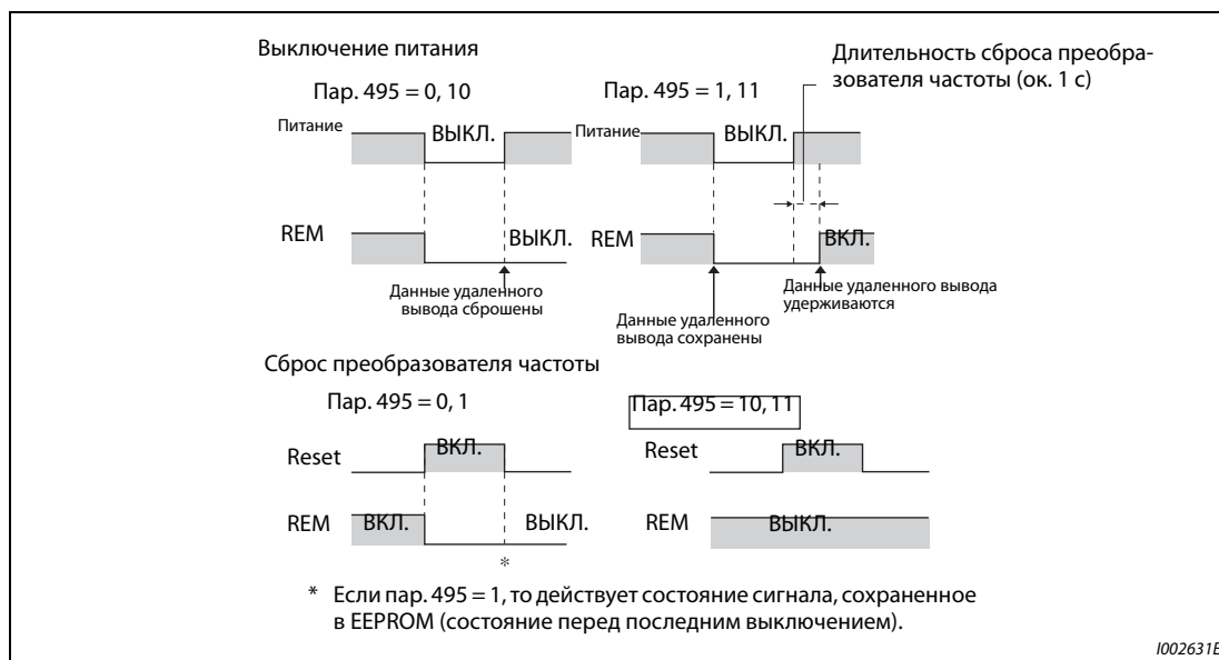
Рис. 5-105: Данные удаленного вывода при положительной логике
