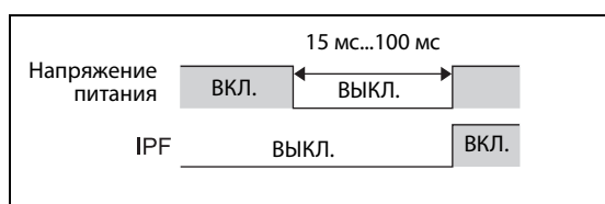
Рис. 5-204: Сигнал IPF
