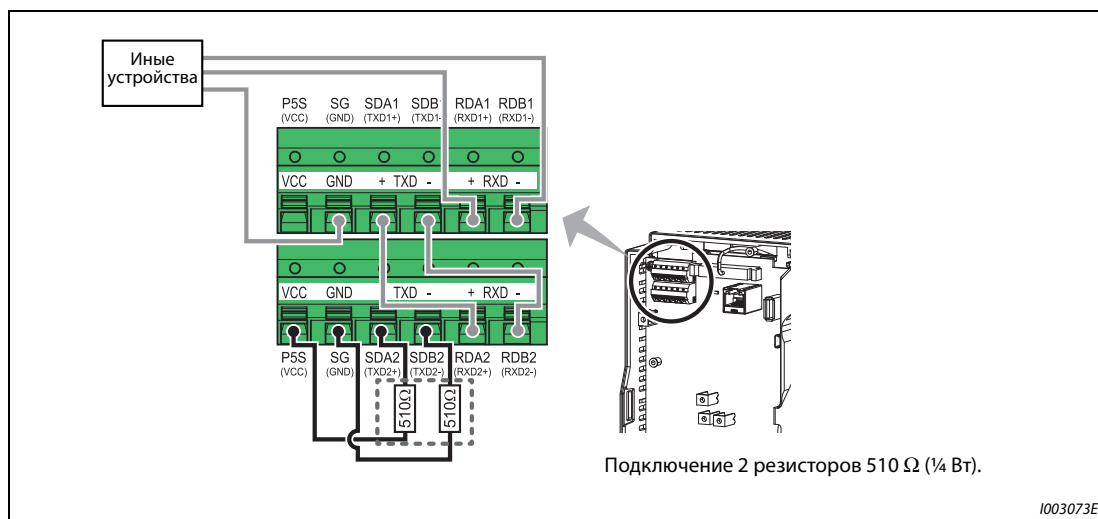
Рис. 5-246: Подключение нагрузочных резисторов к преобразователю частоты
