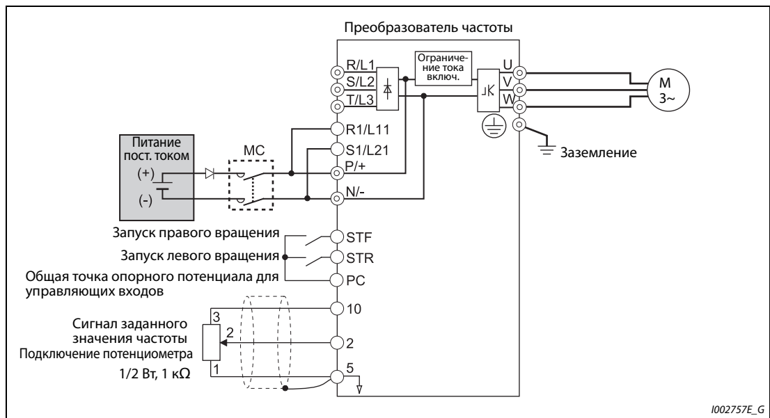
Рис. 5-271: Пример подключения для варианта 1 питания контура постоянного тока
