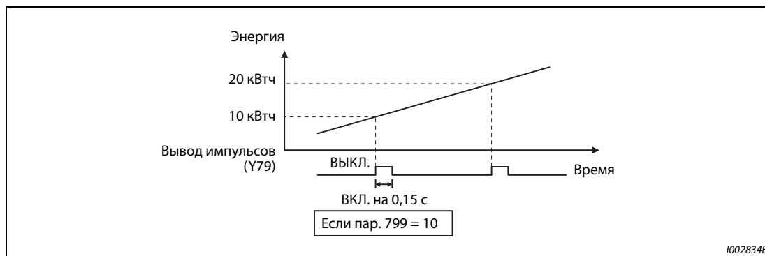
Рис. 5-110: Вывод импульсов энергии
