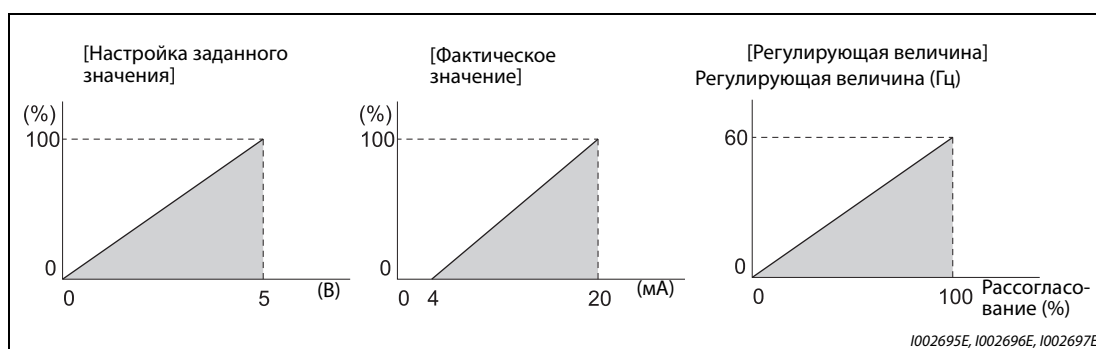
Рис. 5-174: Калибровка входов
