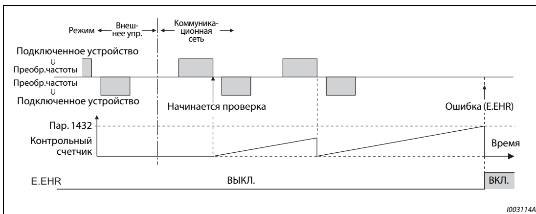
Рис. 5-255: Временная диаграмма контроля коммуникации (Ethernet)
