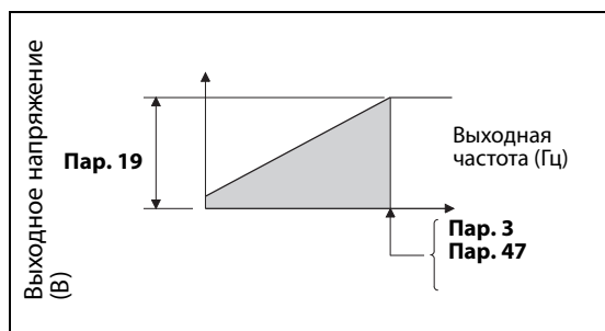
Рис. 5-260: Соотношение выходного напряжения и выходной частоты
