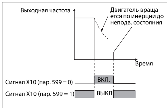
Рис. 5-270: Сигнал X10
