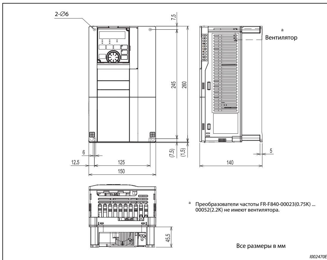
Рис. 8-5: Габаритно-присоединительные размеры преобразователей частоты FR-F820-00105(2.2K), 00167(3.7K), 00250(5.5K), FR-F840-00023(0.75K), 00038(1.5K), 00052(2.2K), 00083(3.7K), 00126(5.5K)
