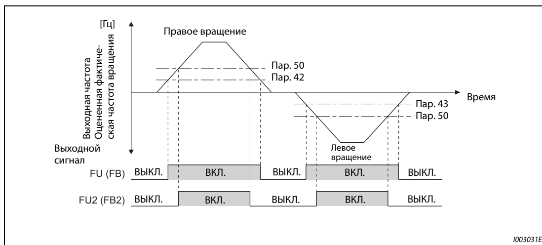
Рис. 5-98: Контроль частоты при правом и левом вращении
