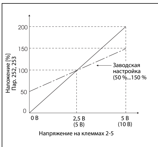
Рис. 5-121: Процентное наложение
