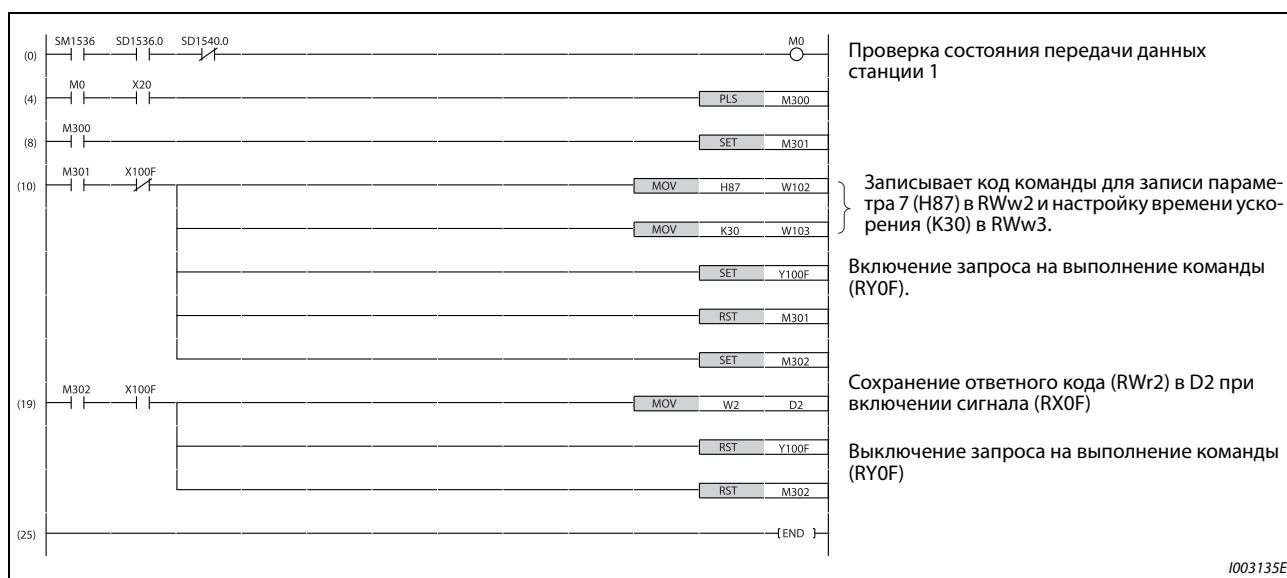
Рис. 5-295: Пример программы 6
