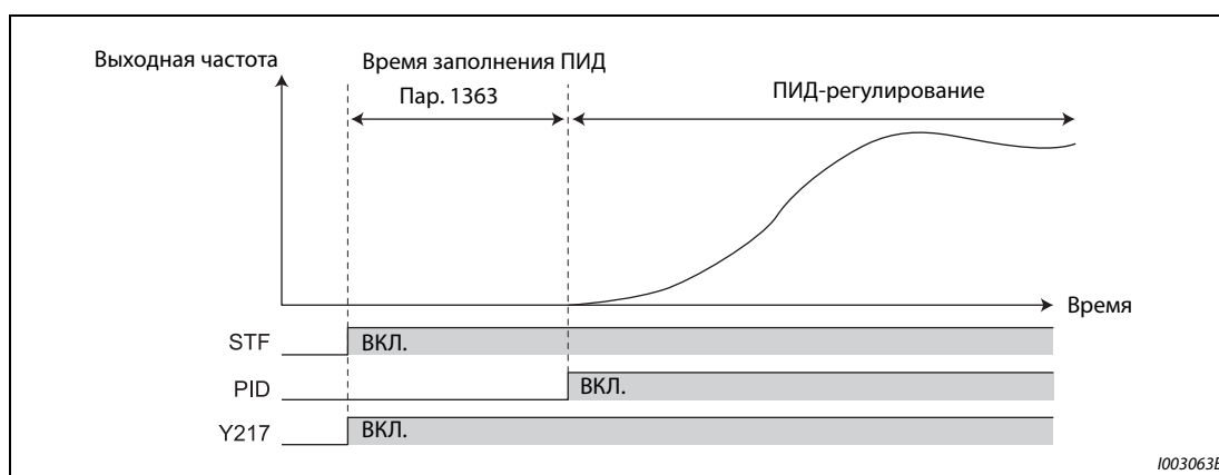
Рис. 5-197: Режим заполнения
