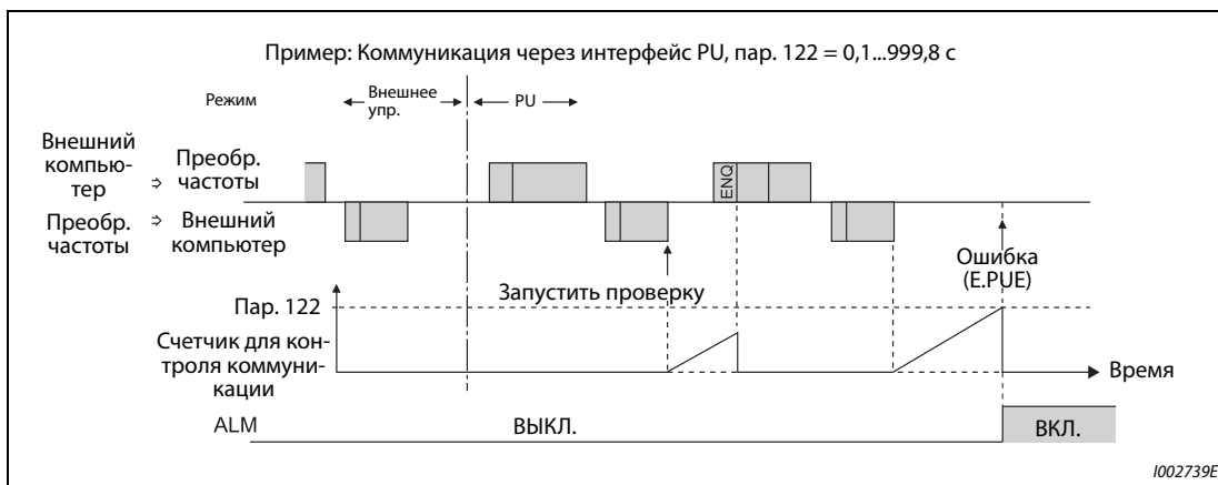
Рис. 5-240: Контроль на обрыв кабеля
