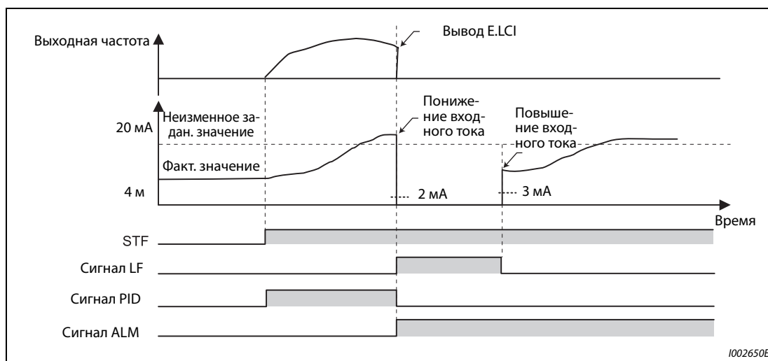
Рис. 5-130: Сообщение о неполадке (пар. 573 = 2)
