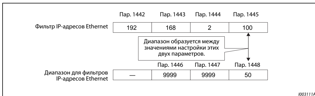
Рис. 5-252: Пример 2 настройки для фильтрации IP-адресов Ethernet
