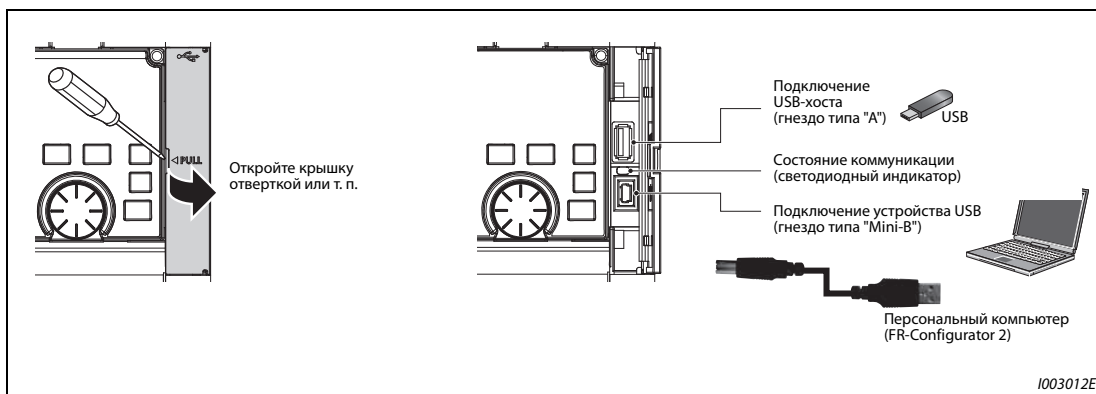
Рис. 2-46: Соединения USB
