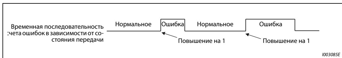
Рис. 5-234: Счет ошибок коммуникации
