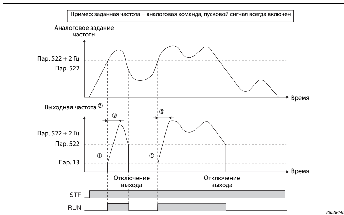
Рис. 5-267: Пример отключения выхода
