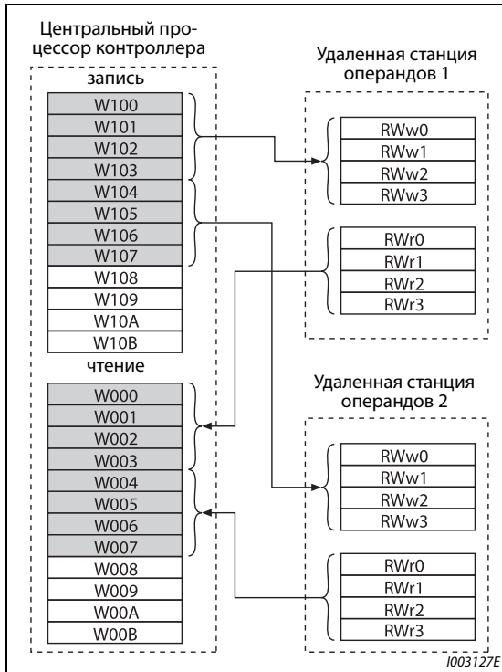
Рис. 5-289: Удаленные регистры
