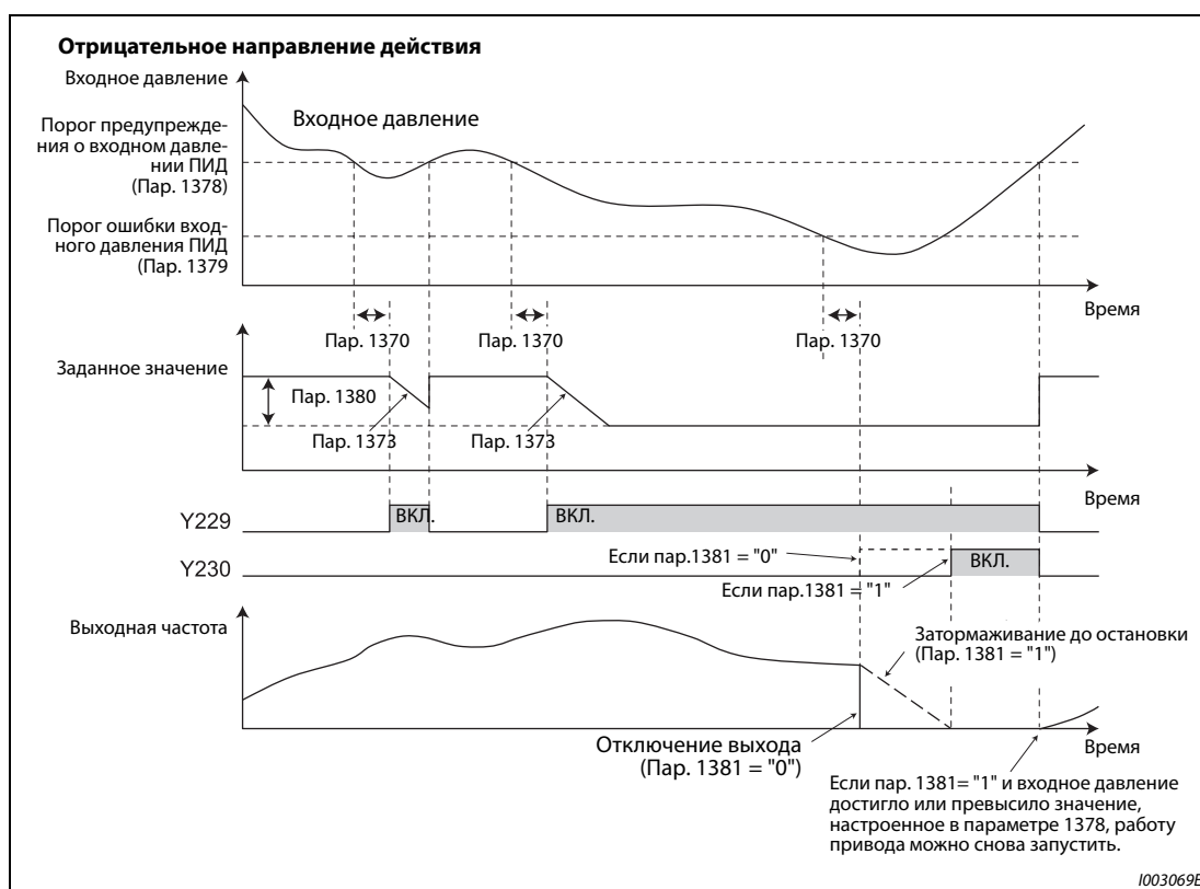
Рис. 5-203: PID-регулирование входного давления
