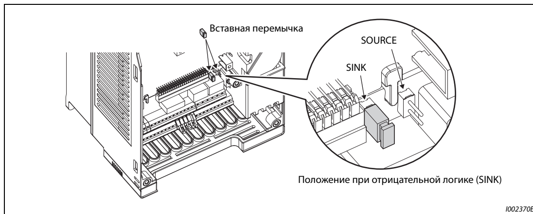
Рис. 2-26: Изменение управляющей логики
