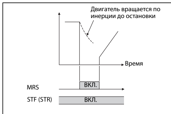
Рис. 5-134: Блокировка регулятора
