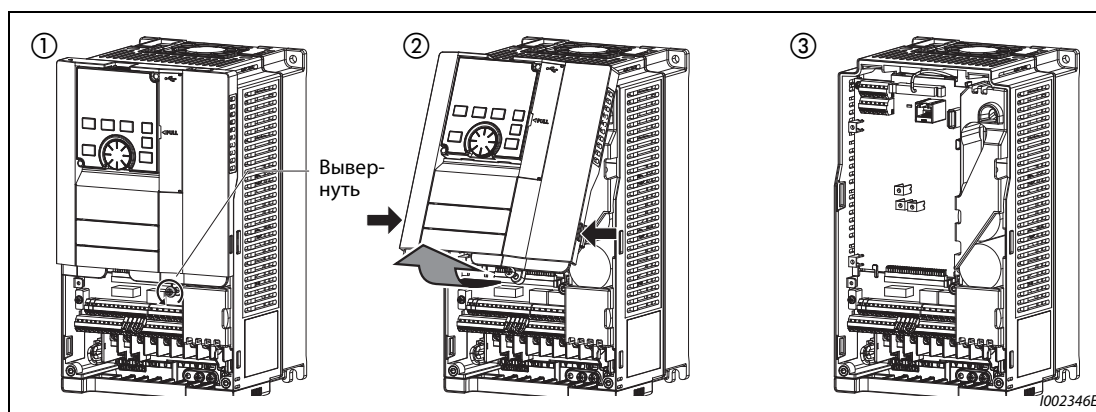
Рис. 2-8: Снятие верхней передней панели
