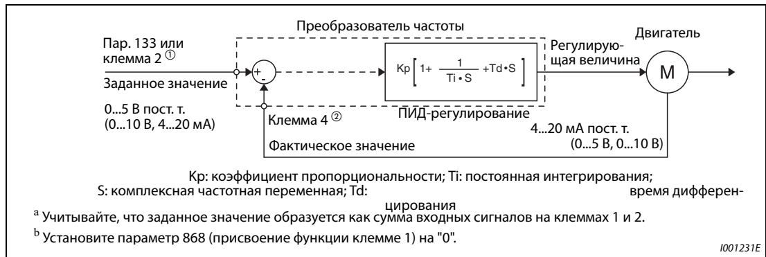
Рис. 5-160: Конфигурация системы для пар. 128 = 20 или 21 (подключение задания/сигнала обратной связи к преобразователю)
