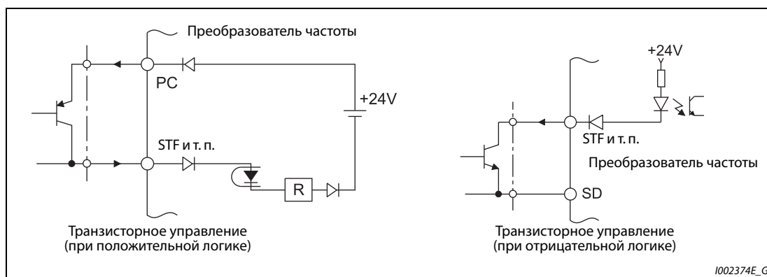
Рис. 2-36: Управление входами через транзисторы
