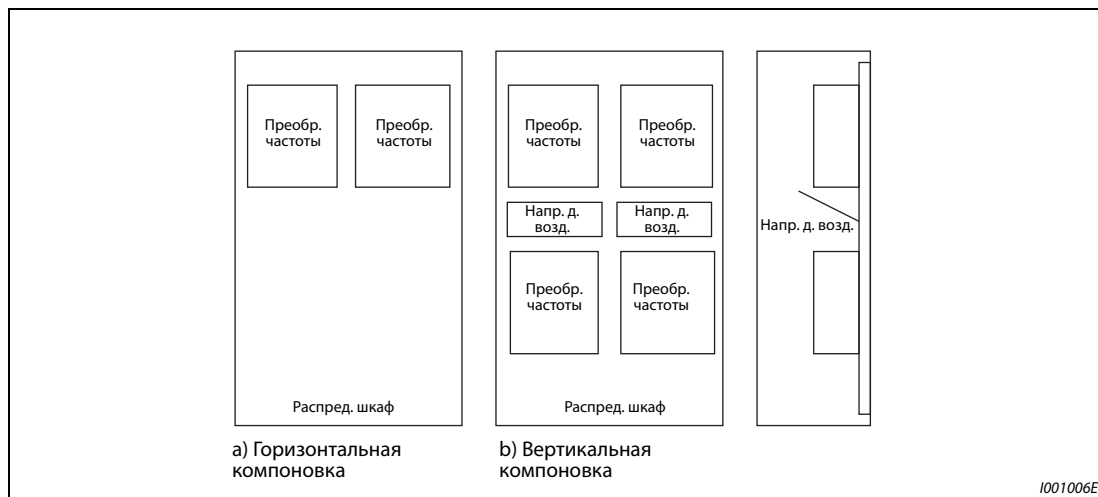
Рис. 2-15: Компоновка в случае установки нескольких преобразователей
