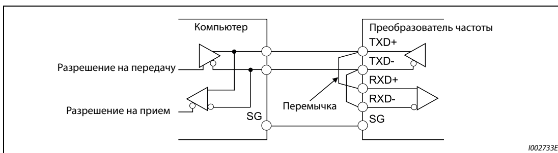
Рис. 5-230: Соединение по 2-проводной схеме
