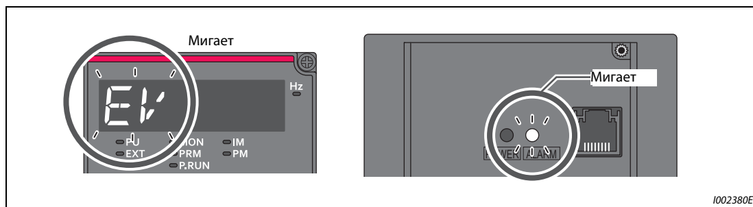
Рис. 2-43: Признаки внешнего питания контура управления
