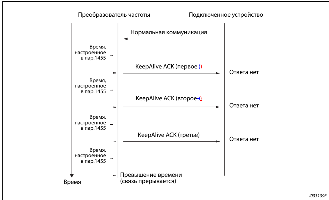
Рис. 5-250: Процесс проверки поддержания связи
