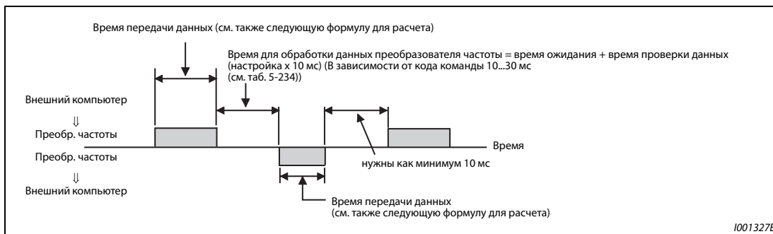
Рис. 5-238: Время передачи
