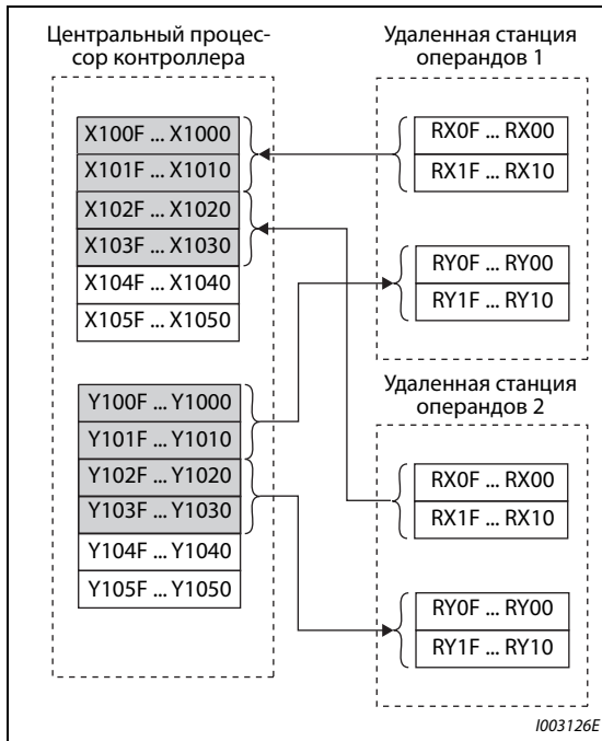
Рис. 5-288: Децентрализованный ввод-вывод
