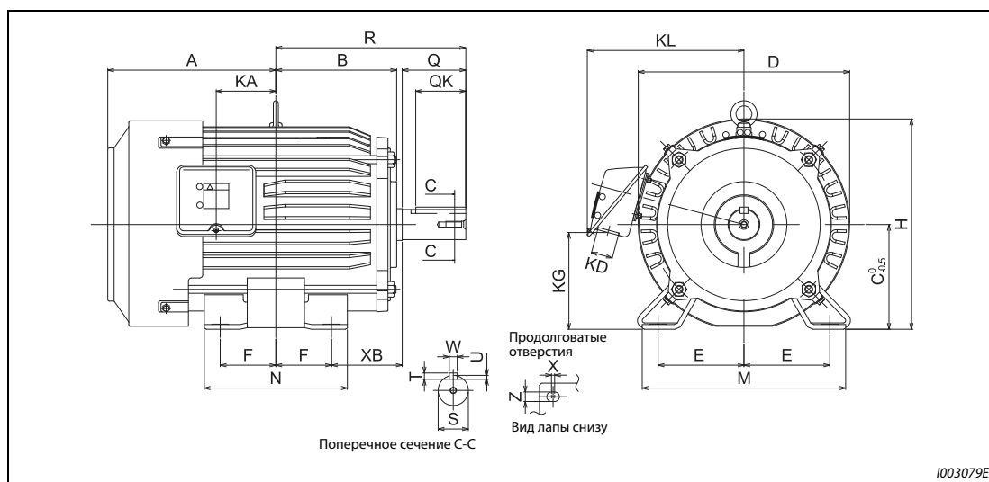
Рис. 8-15: Габаритно-присоединительные размеры MM-EFS (ном. частота вращения 3000 мин -1 )
