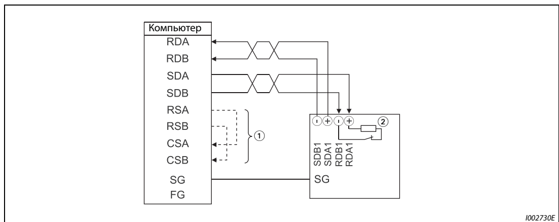
Рис. 5-228: Соединение с одним преобразователем частоты
