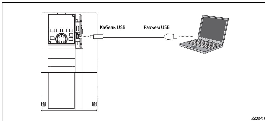
Рис. 5-257: Подключение к интерфейсу USB
