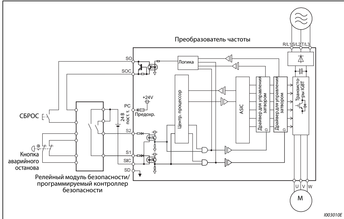
Рис. 2-44: Подключение релейного модуля безопасности
