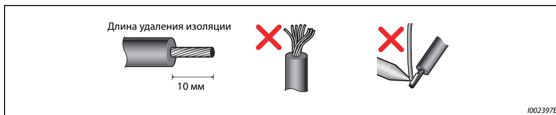
Рис. 2-31: Подготовка провода
