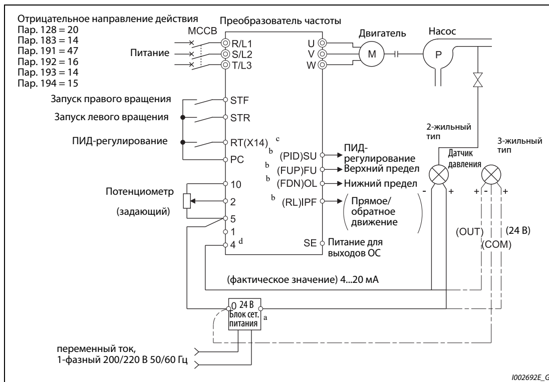
Рис. 5-166: Пример подключения по положительной логике
