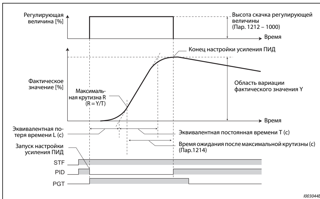
Рис. 5-175: Временная последовательность при методе реакции на скачок
