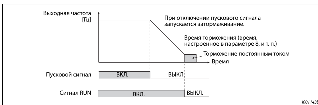
Рис. 5-268: Метод останова, если параметр 250 = 8888 или 9999
