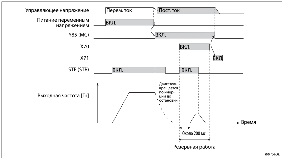
Рис. 5-273: Пример 1 работы при исчезновении сетевого напряжения
