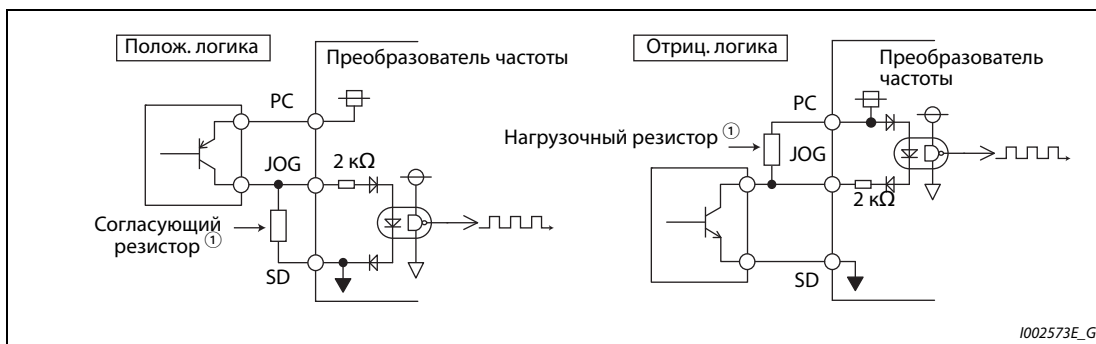
Рис. 5-37: Импульсный вход
