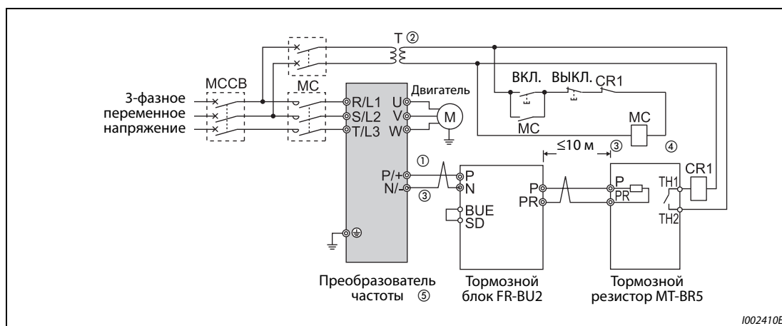
Рис. 2-50: Подключение тормозного блока с тормозным резистором MT-BR5
