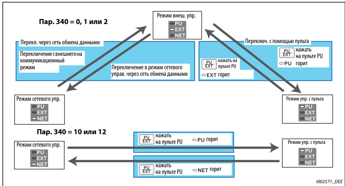
Рис. 5-32: Переключение режима
