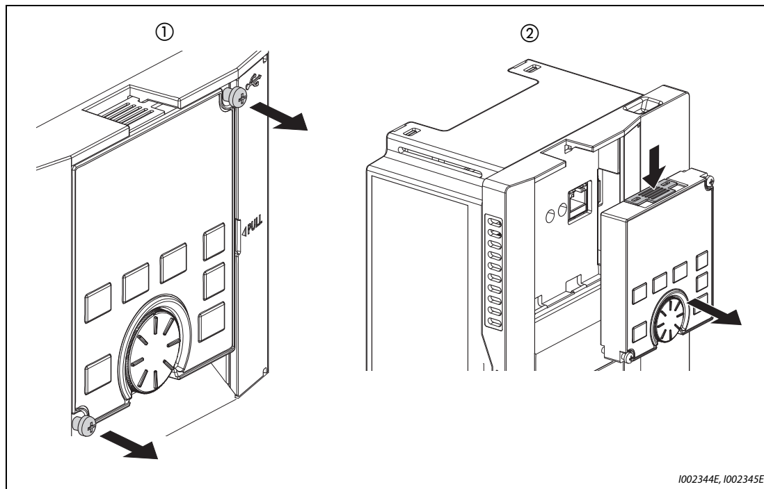
Рис. 2-6: Снятие и установка пульта
