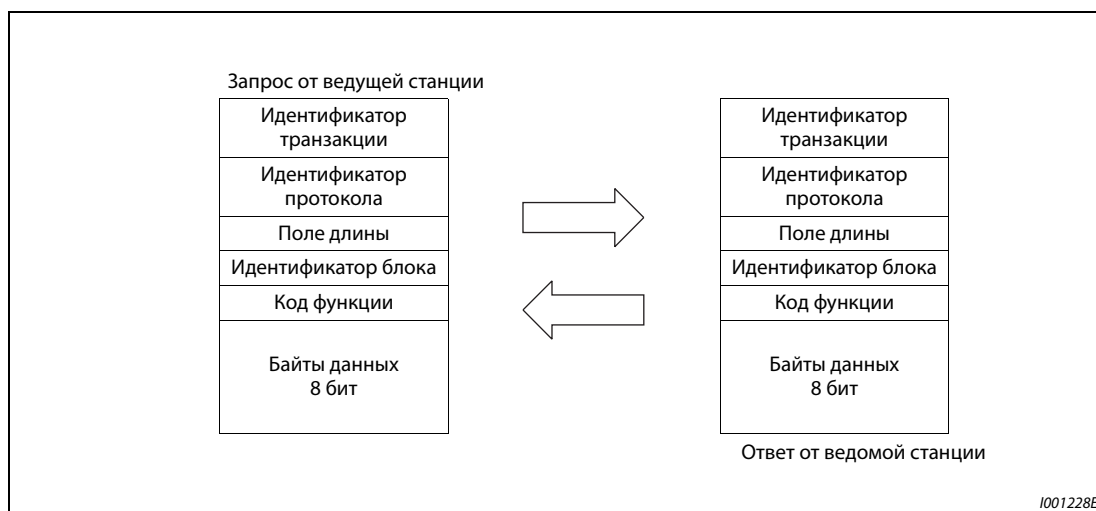
Рис. 5-286: Обмен данными
