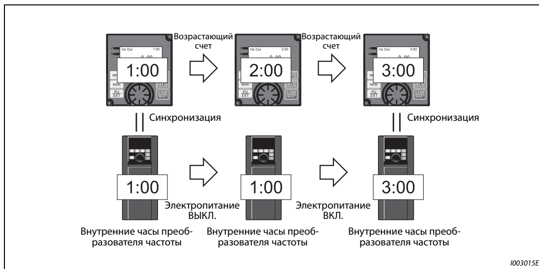
Рис. 5-7: Синхронизация внутренних часов с часами FR-LU08
