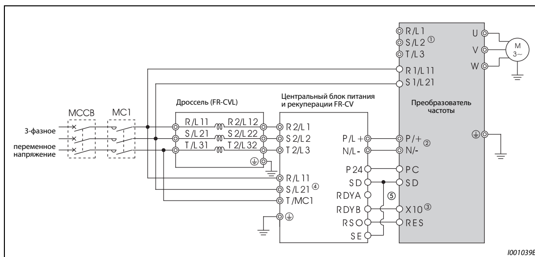
Рис. 2-54: Подключение центрального блока питания и рекуперации FR-CV
