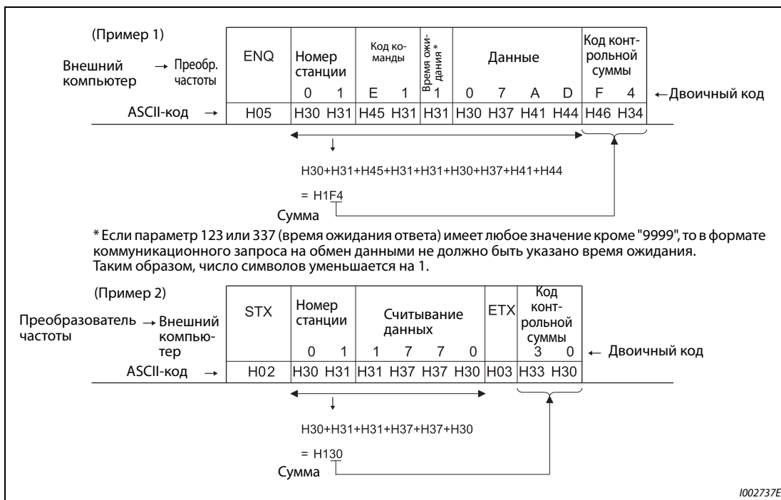
Рис. 5-237: Код контрольной суммы (примеры)
