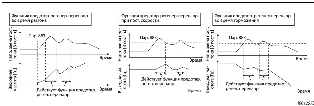
Рис. 5-276: Функция предотвращения регенеративного перенапряжения
