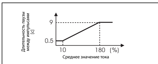
Рис. 5-14: Длительность паузы между импульсами, отображающей среднее значение тока
