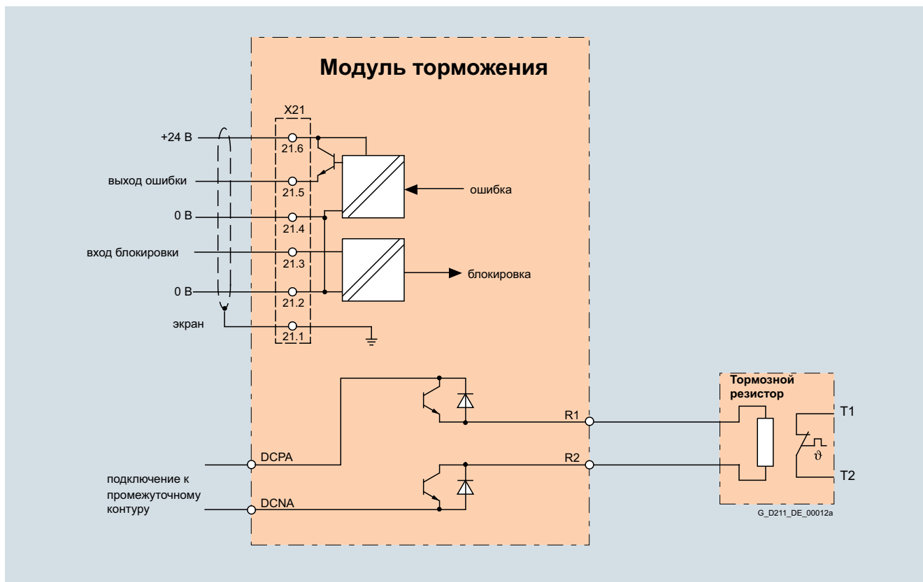
Пример подключения модуля торможения
