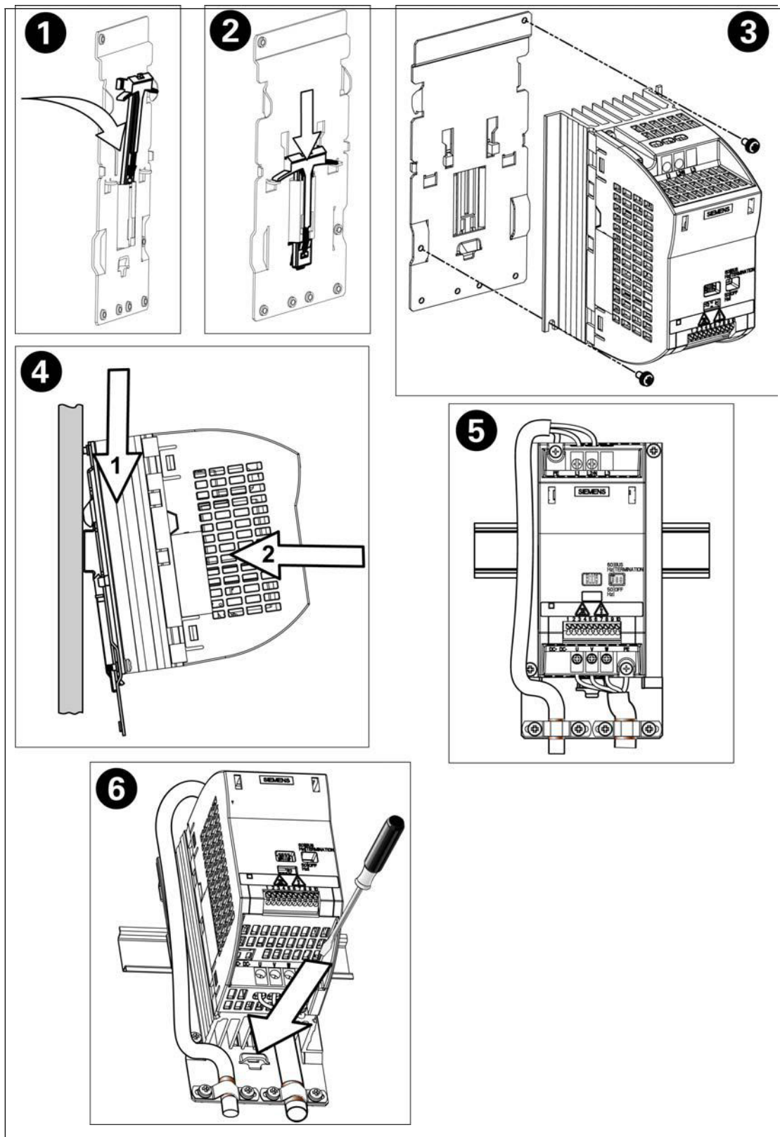
Рис. В-1 Установка статического преобразователя с помощью адаптера колпачковой шины
