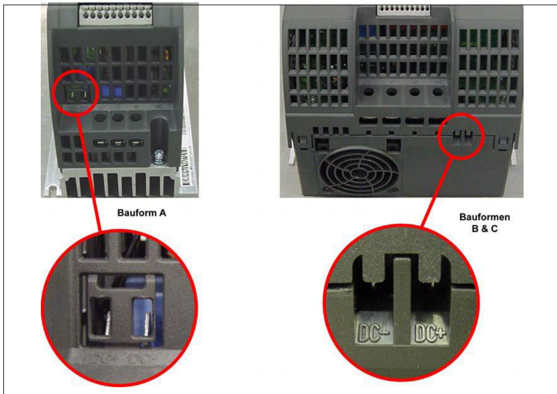
Рис. 2-6 Подключения SINAMICS G110-DC
