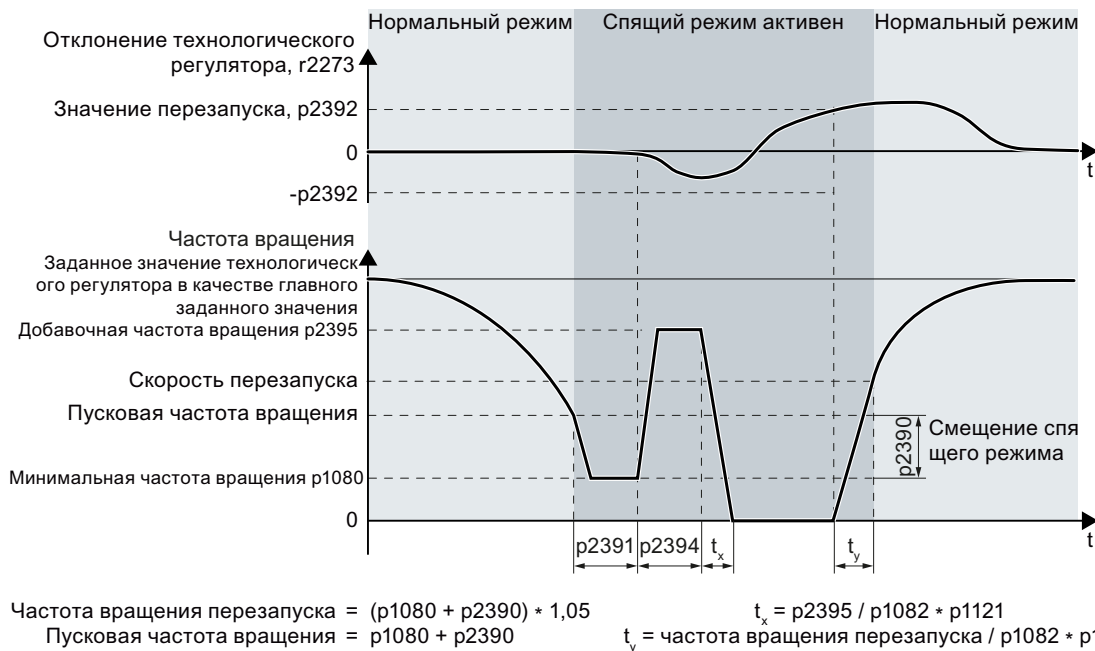
Рис. 8-37 Спящий режим через технологическое заданное значение как главное заданное значение с усилением
