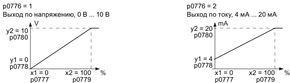
Рис. 6-3 Примеры нормирующих характеристик
