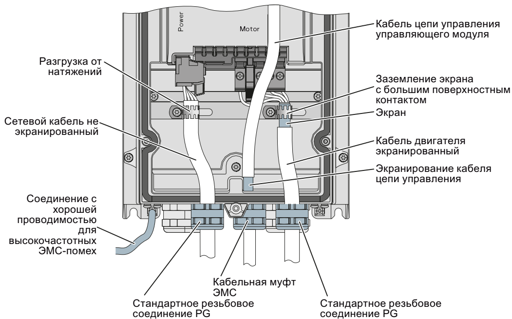
Рис. 4-14 Подключение силового модуля PM230 согласно требованиям ЭМС, степень защиты IP55 / UL тип 12
