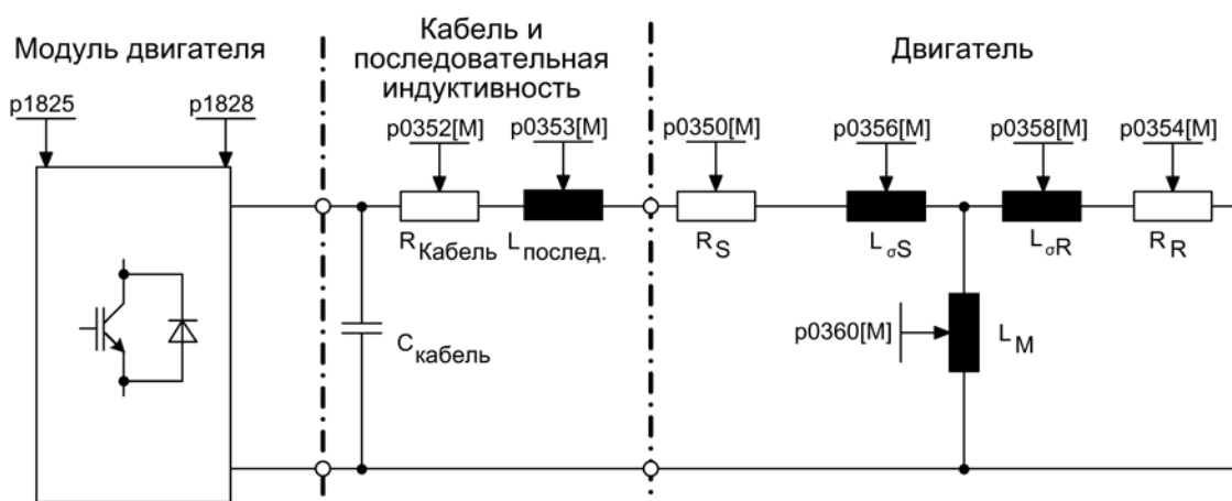
Изображение 3-68 Эквивалентная схема - Асинхронный двигатель и кабель
