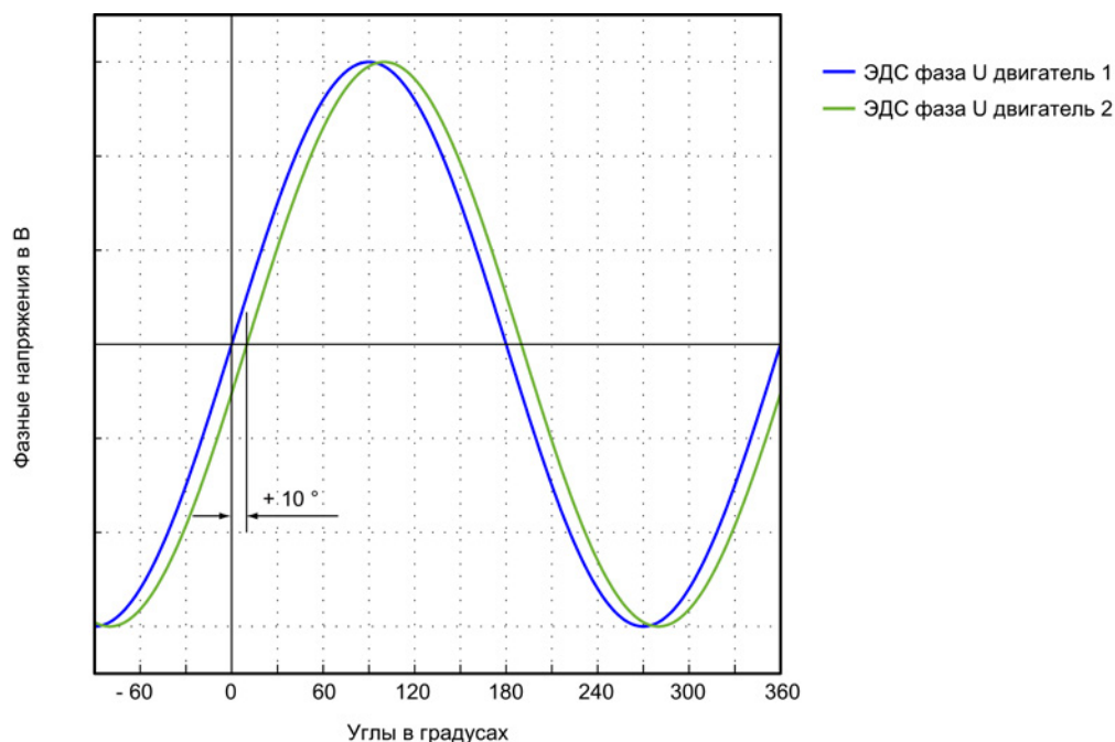
Изображение 3-88 ЭДС фаза U двигателя 1 может опережать ЭДС фаза U двигателя 2 не более чем на 10^\circ
